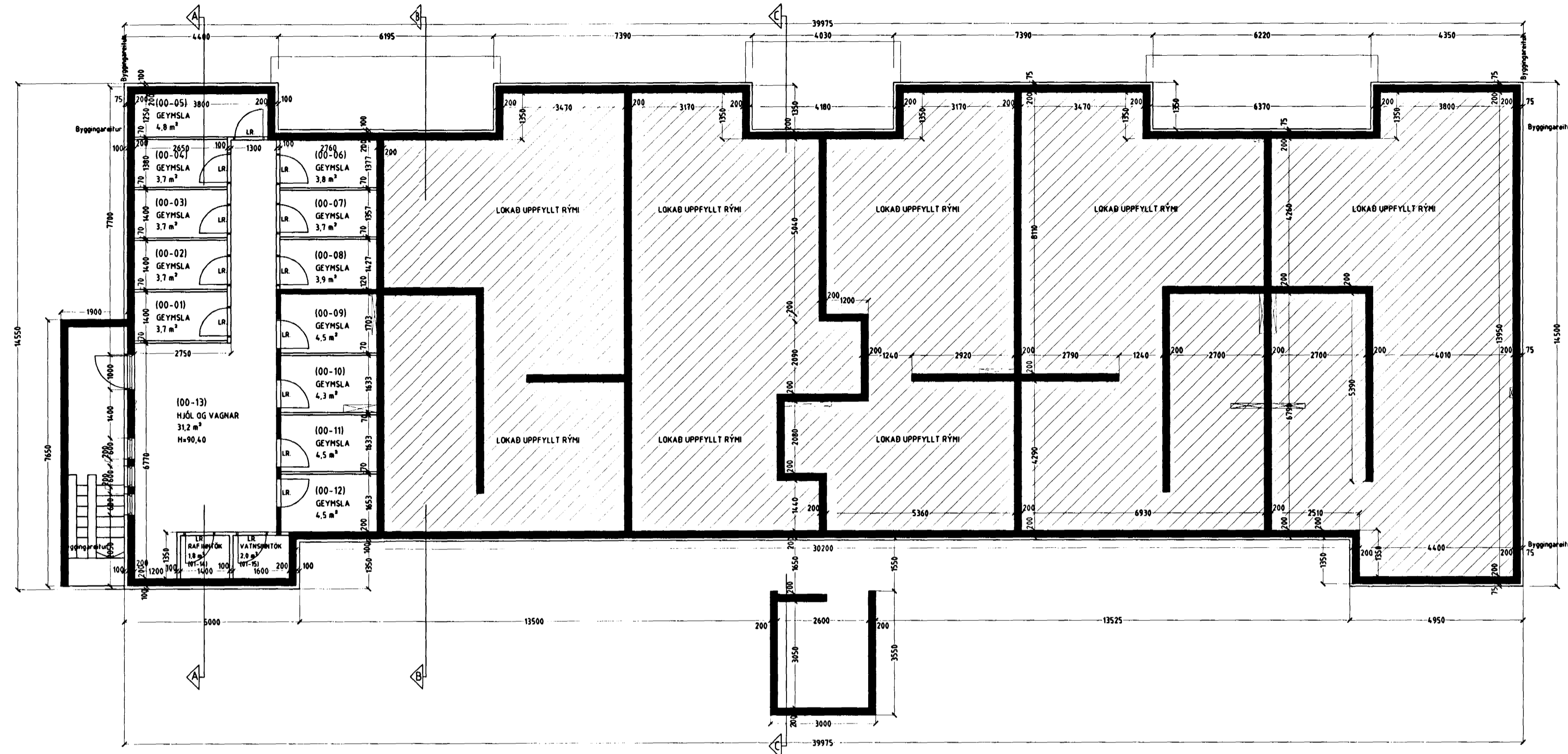
GRUNNMYND JARÐHÆÐ MKV 1:100.
