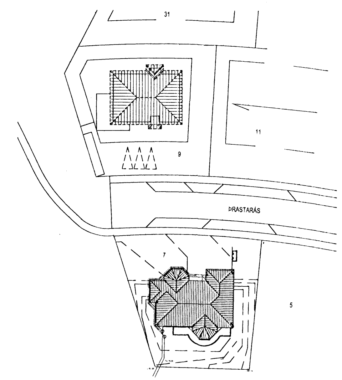
AFSTÖÐUMYND MKV 1:500
