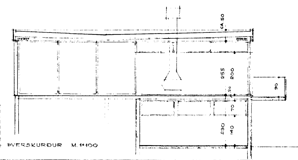
GRUNNMYND KJALLARA M. 1:100
