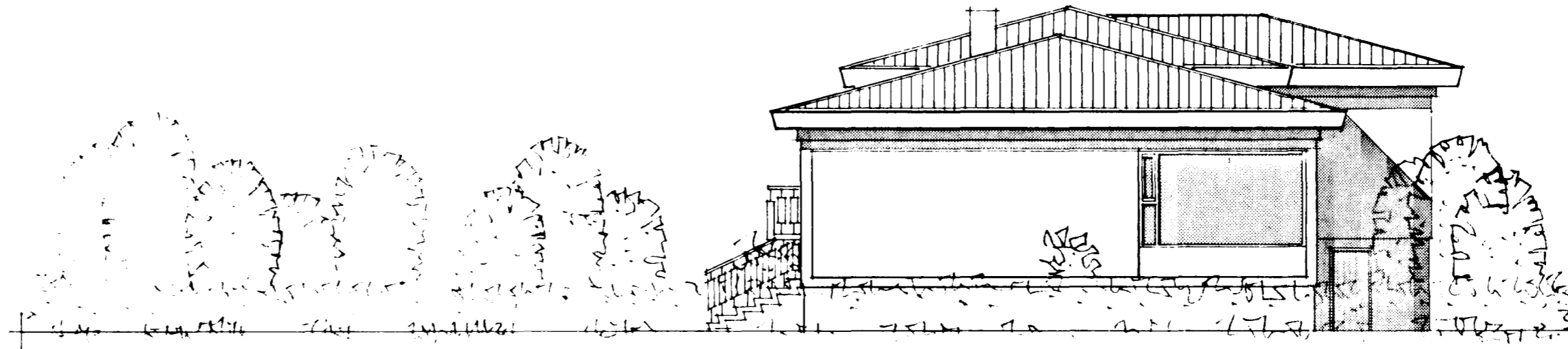
SÚDAUSTUR M.1:100
