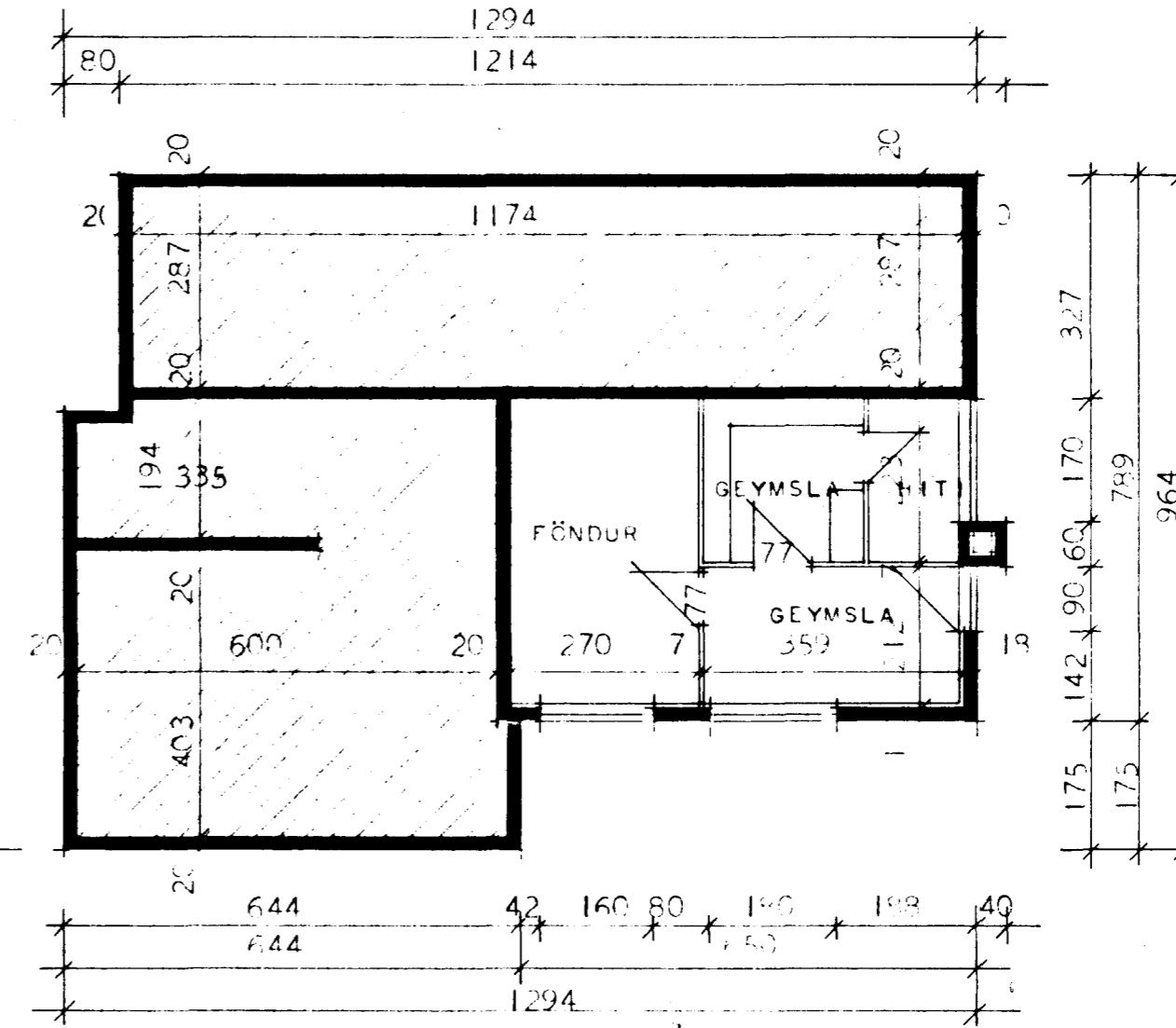
GRUNNMYND KJALLARA NORÐUR
