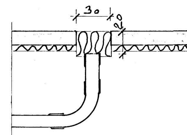
FRÁANGUR STÚTA Í PLÖTU STÚTAR SKULU ENDA 20 cm UNDIR YFIRBORDI OG ÞAR SETT PLAST 30x30 cm.
