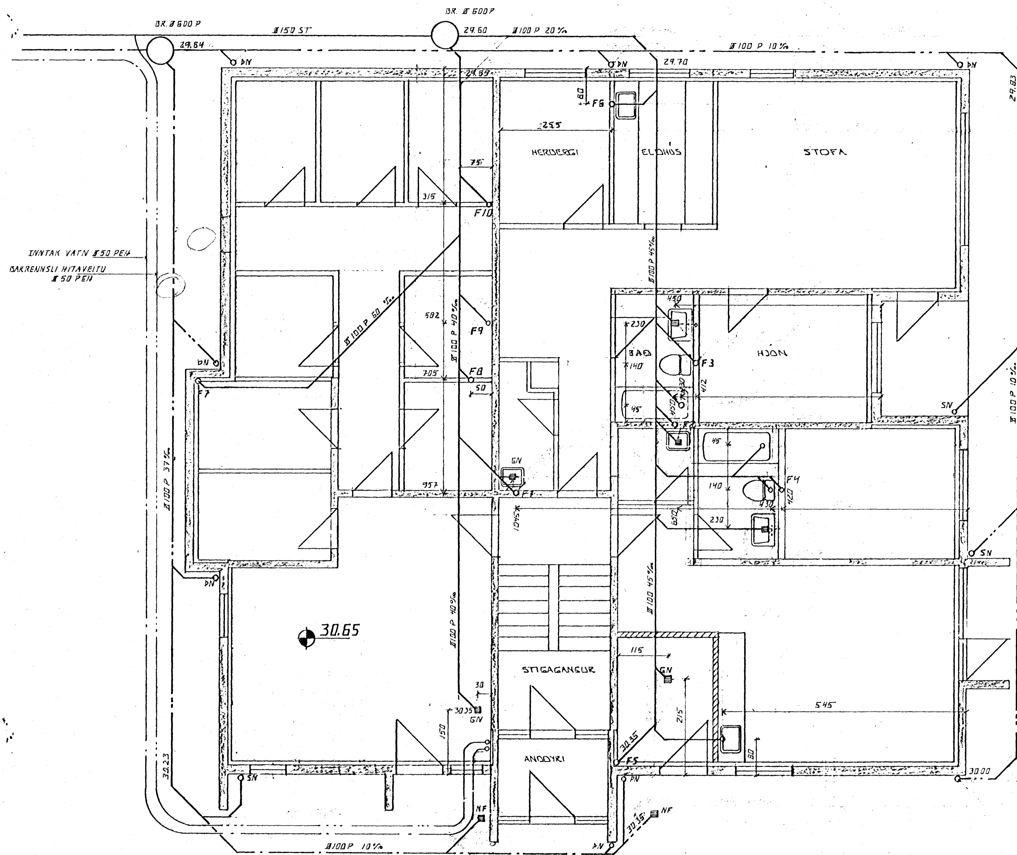
GRUNNMYND • 1:50
