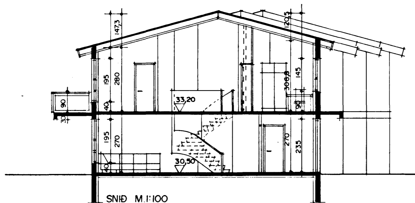
SNIÐ M.1:100
