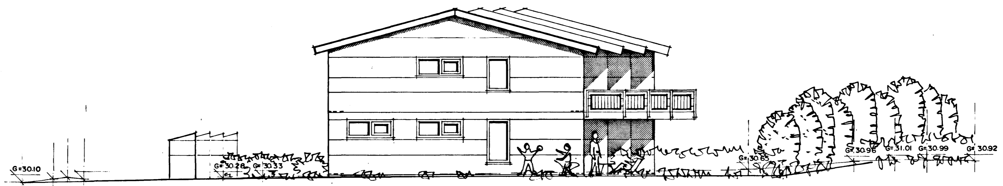
VESTUR M.1:100
