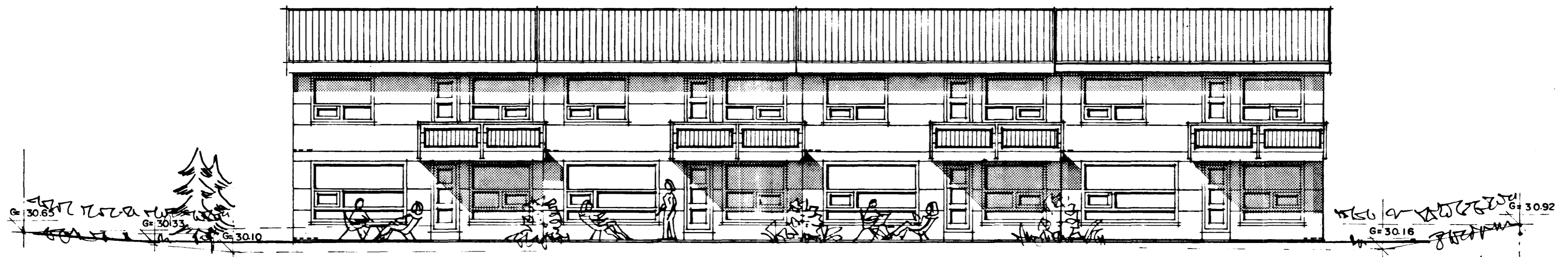
SUDUR M.1:100
