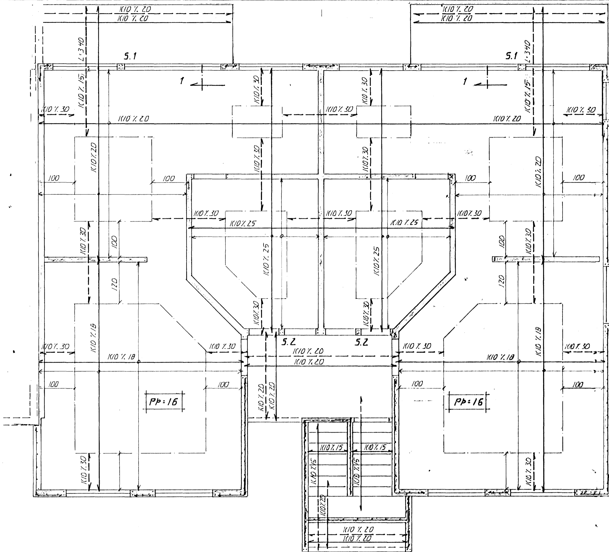
GRUNNMÝND, 1:50
