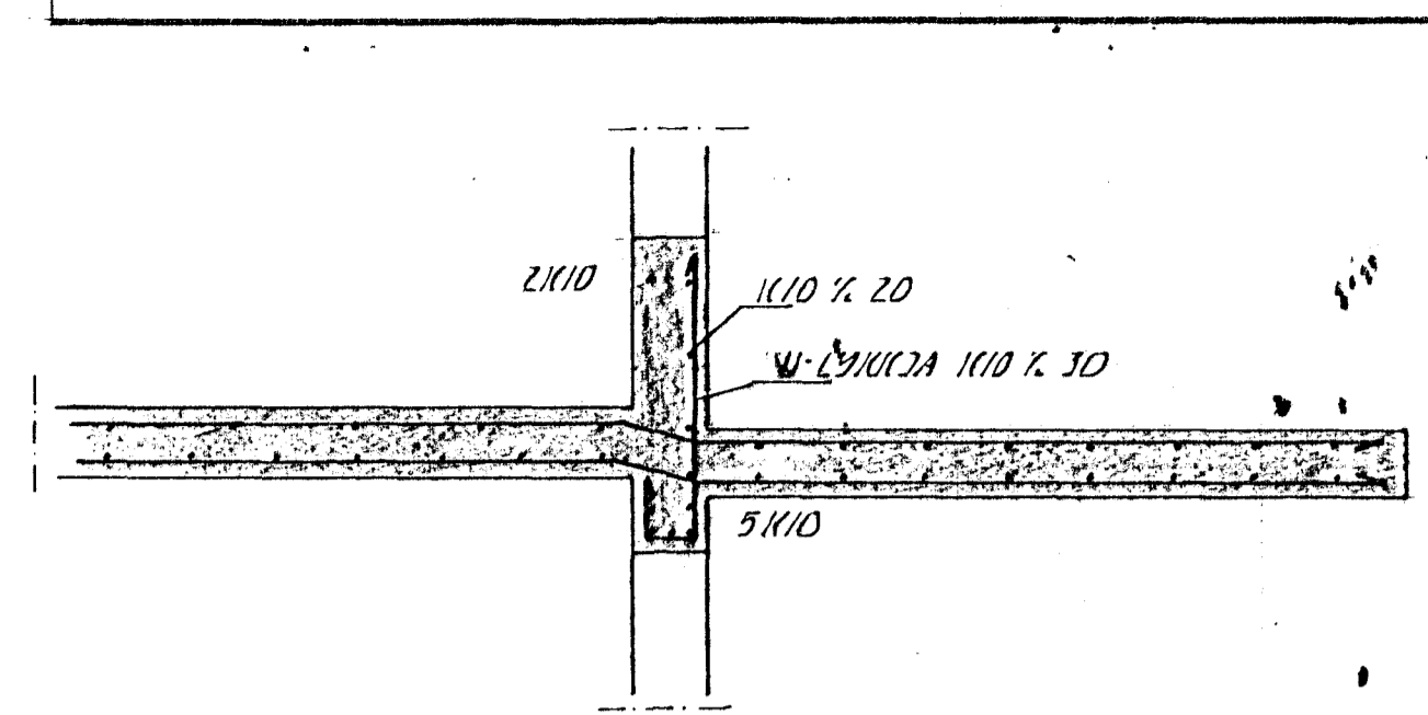
SNIÐ 1. 1:20
