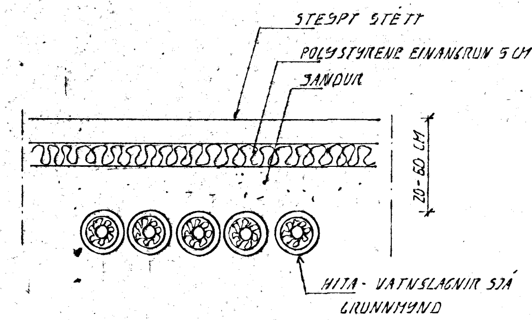
LAGNIR I JÖRD SMÍÐ, 1:10
