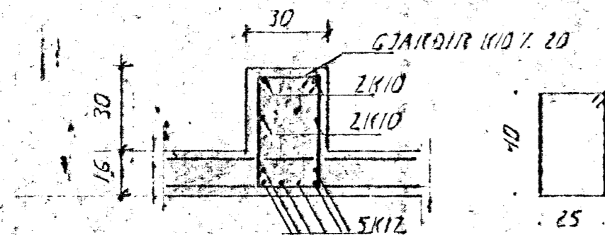
SNID 2. 1:20
