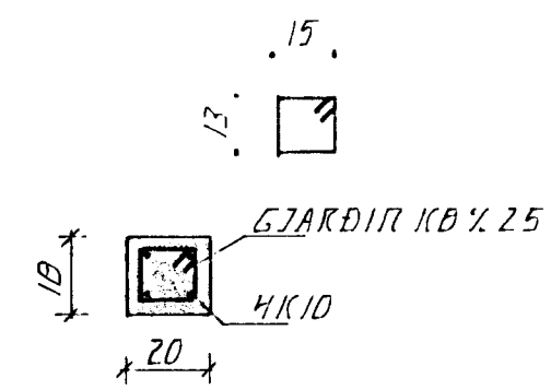
SÚLA 51, 1:20
