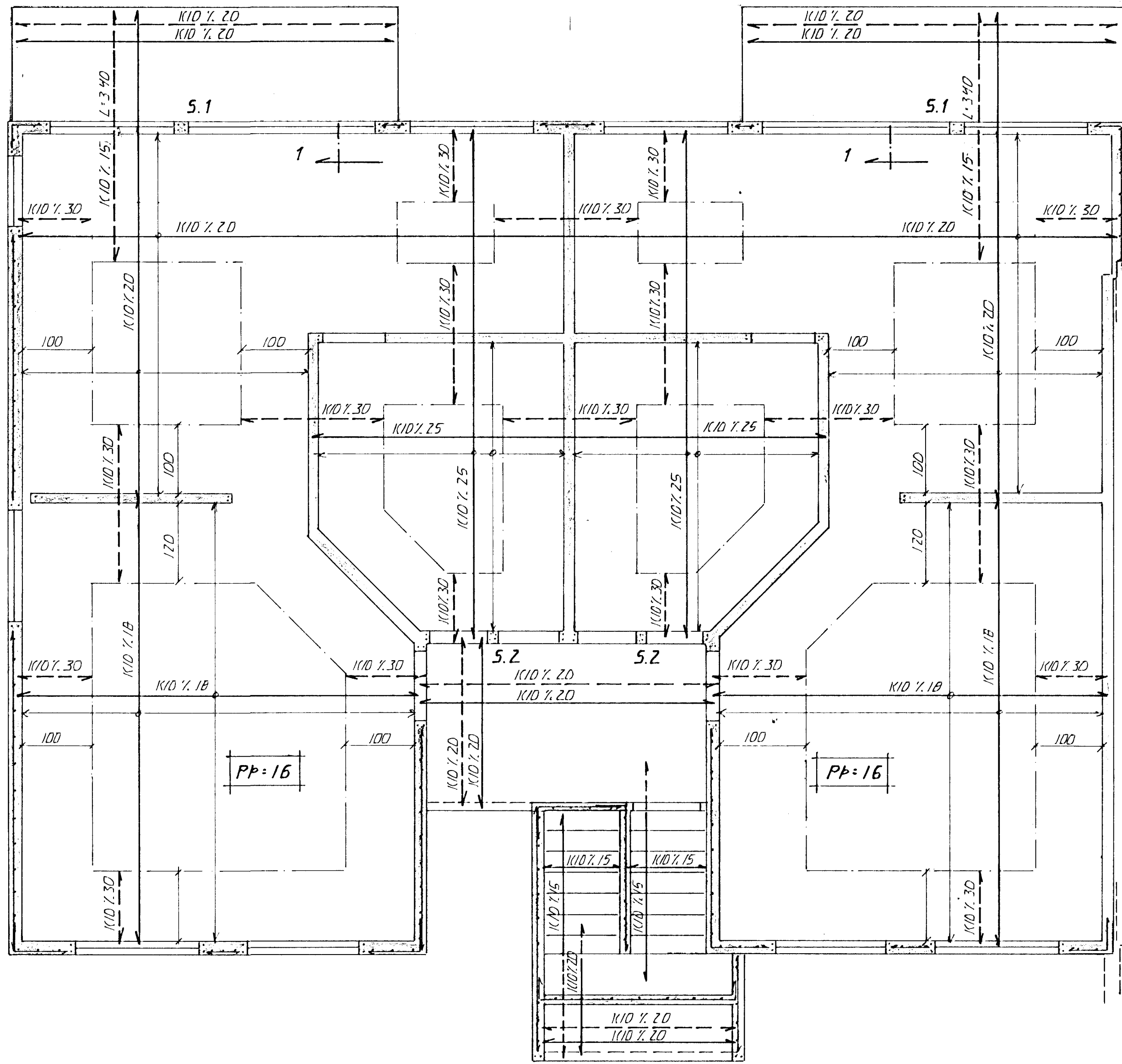
GRUNNMUND, 1:50
