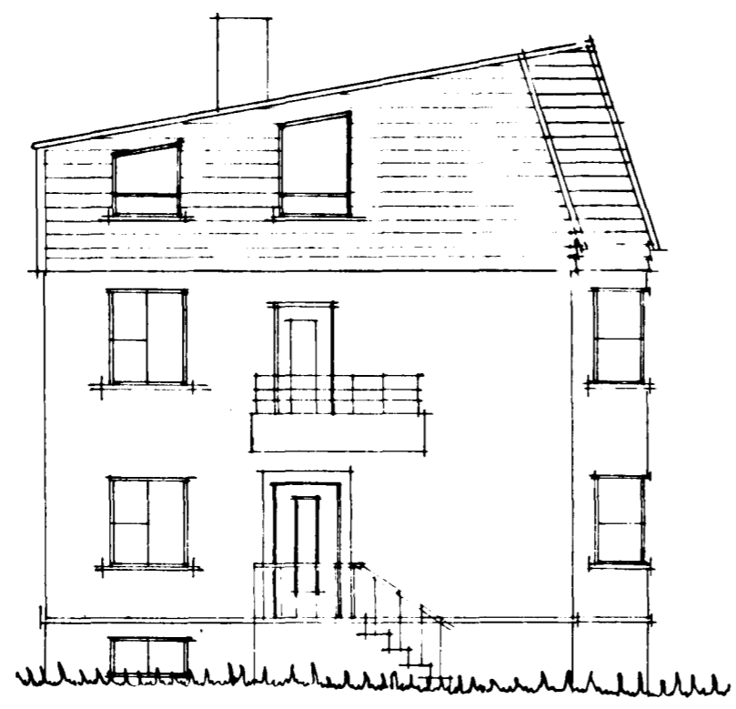
Stafn
