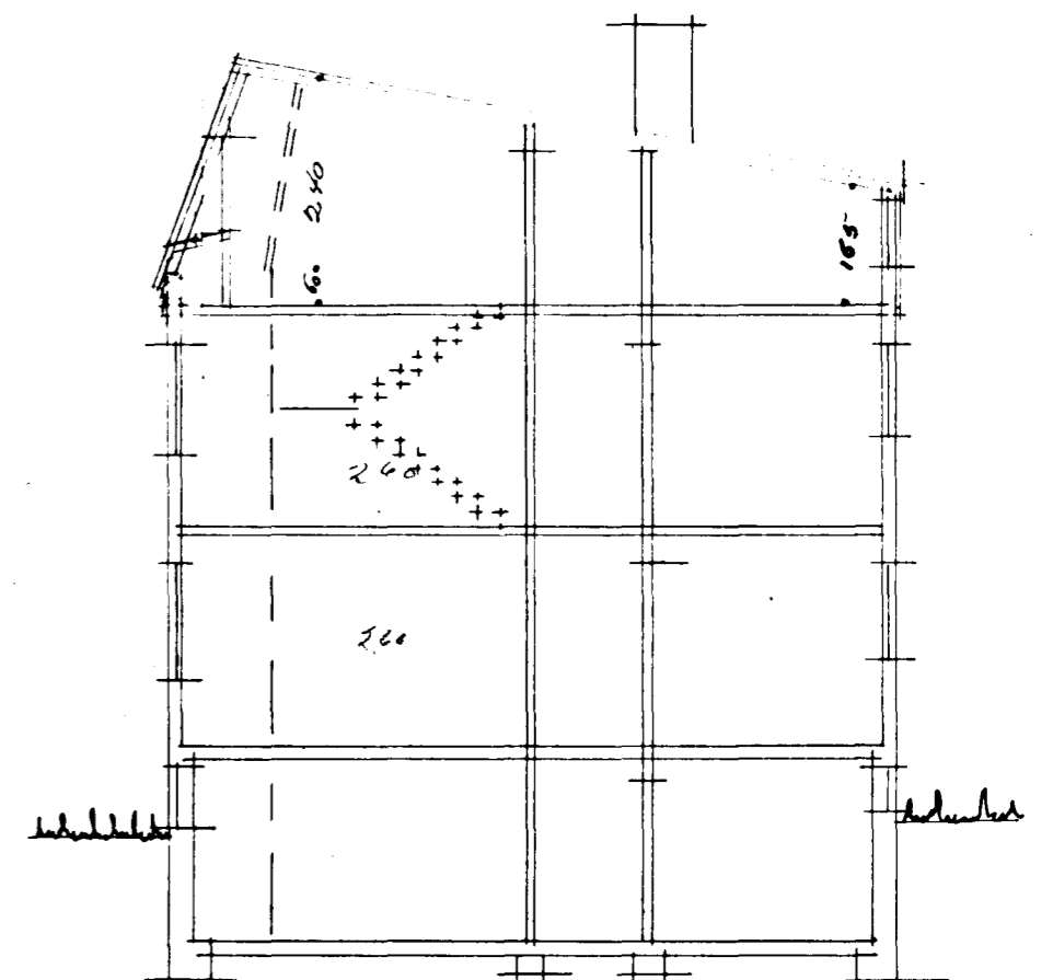
Skurður
