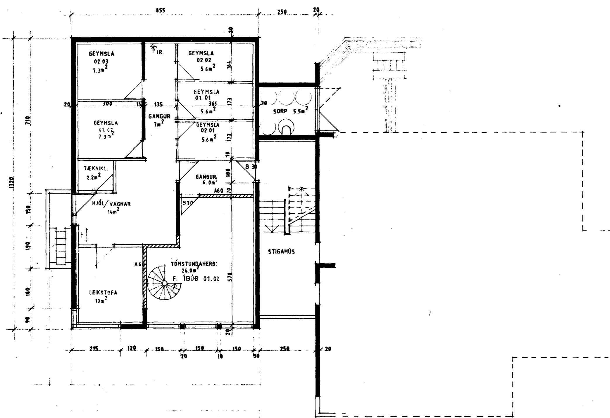
GRUNNMYND KJALLARA
