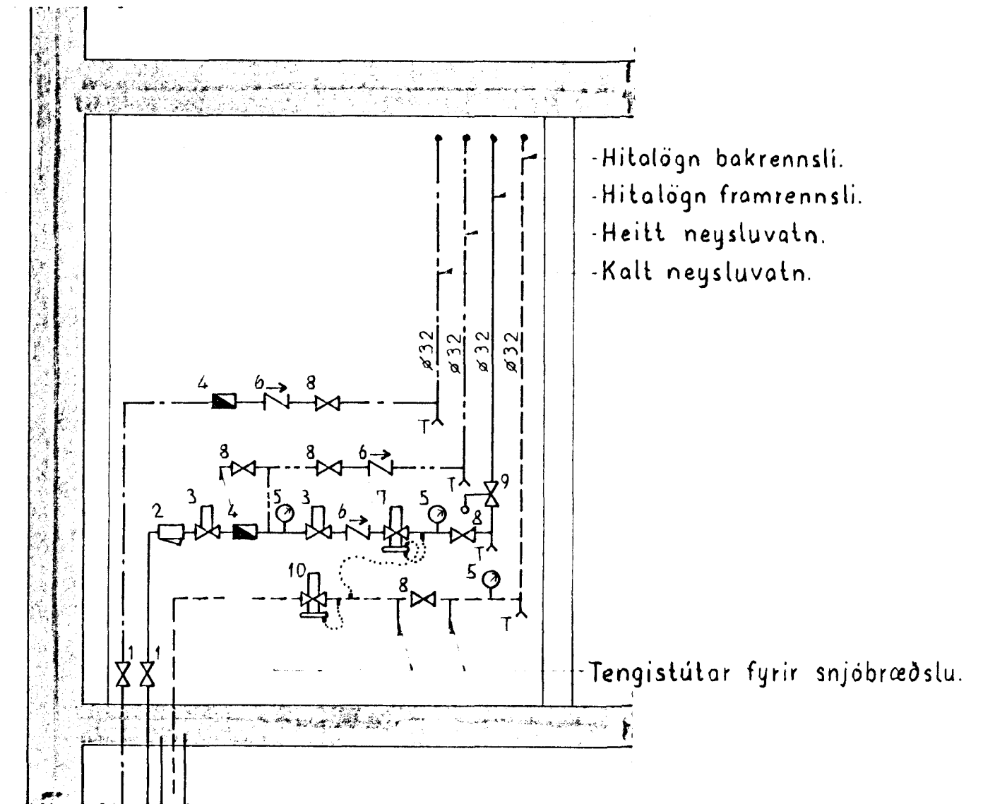
HITAGRIND, 1:20
