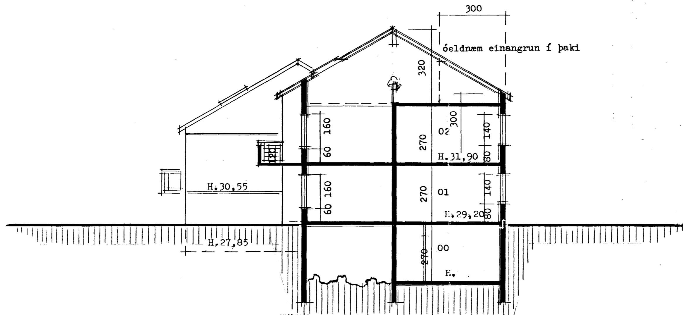
snið b-b
