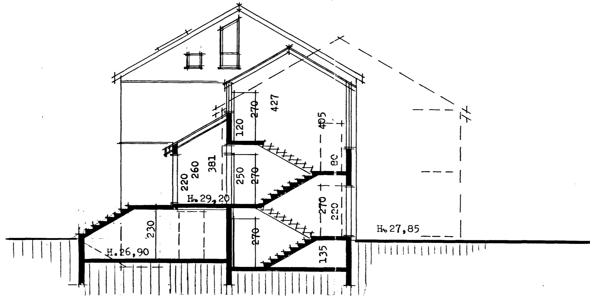
snið a-a
