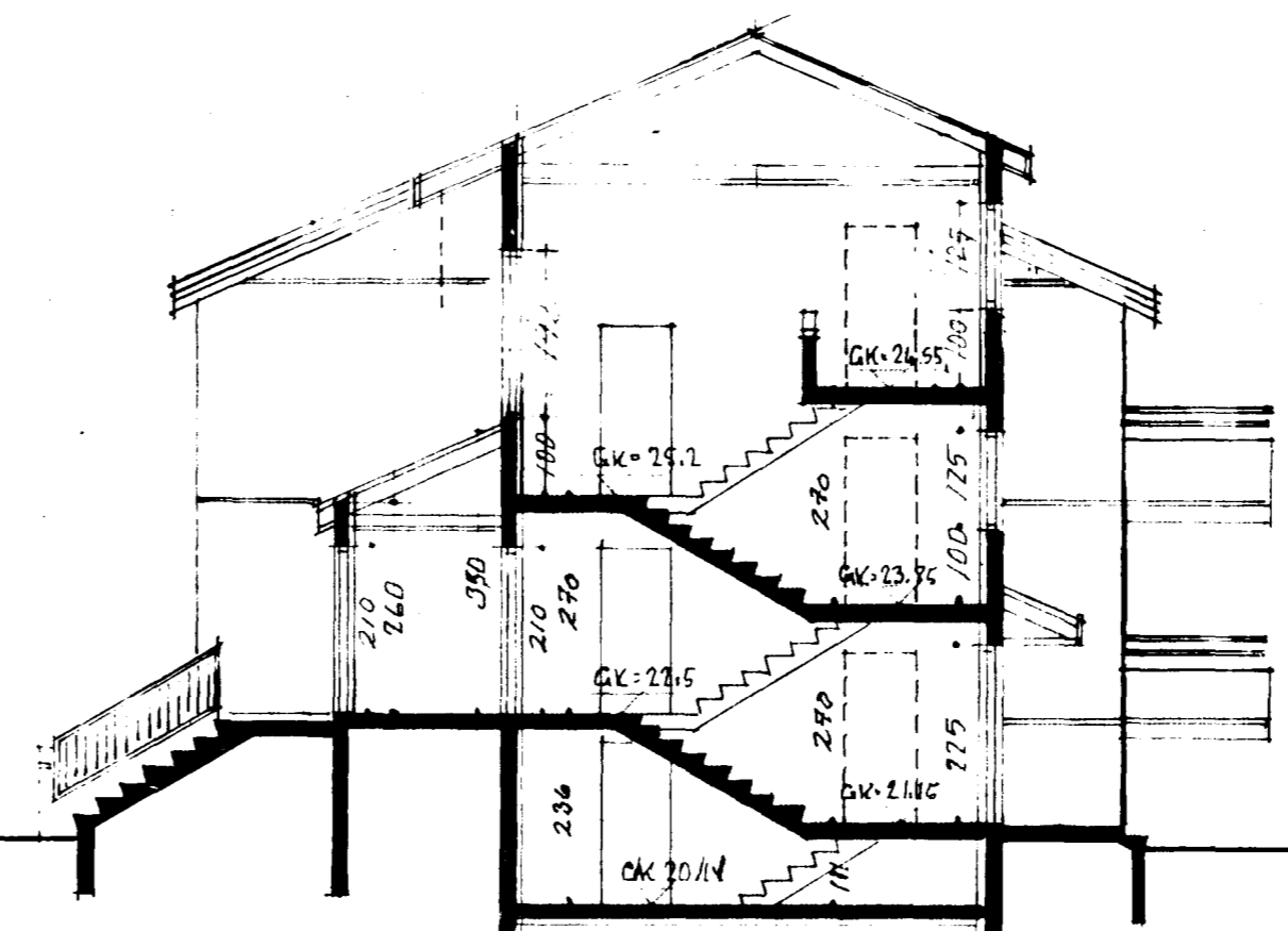
SNID B-B M. 1:100
