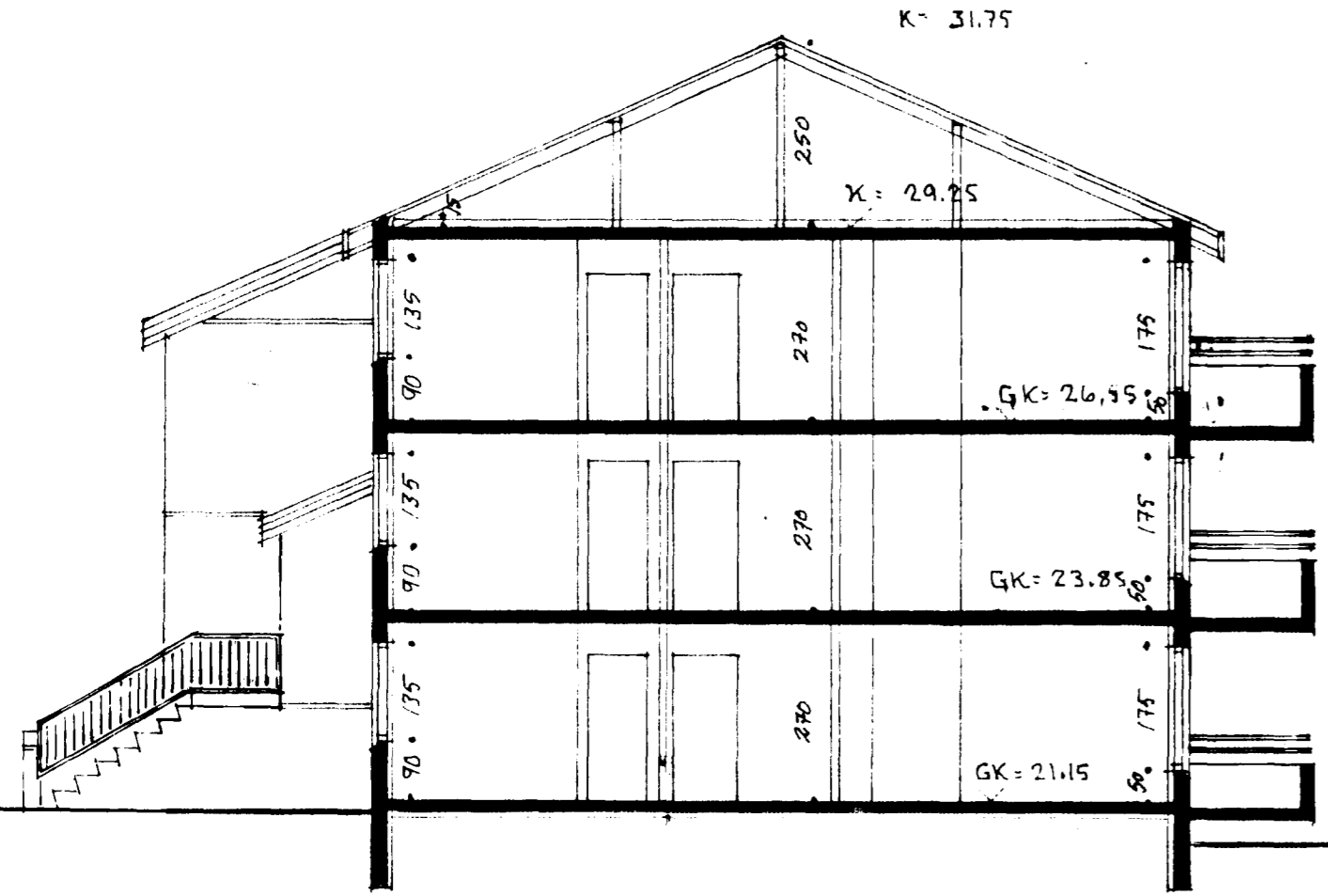
SNID A-A M. 1:100
