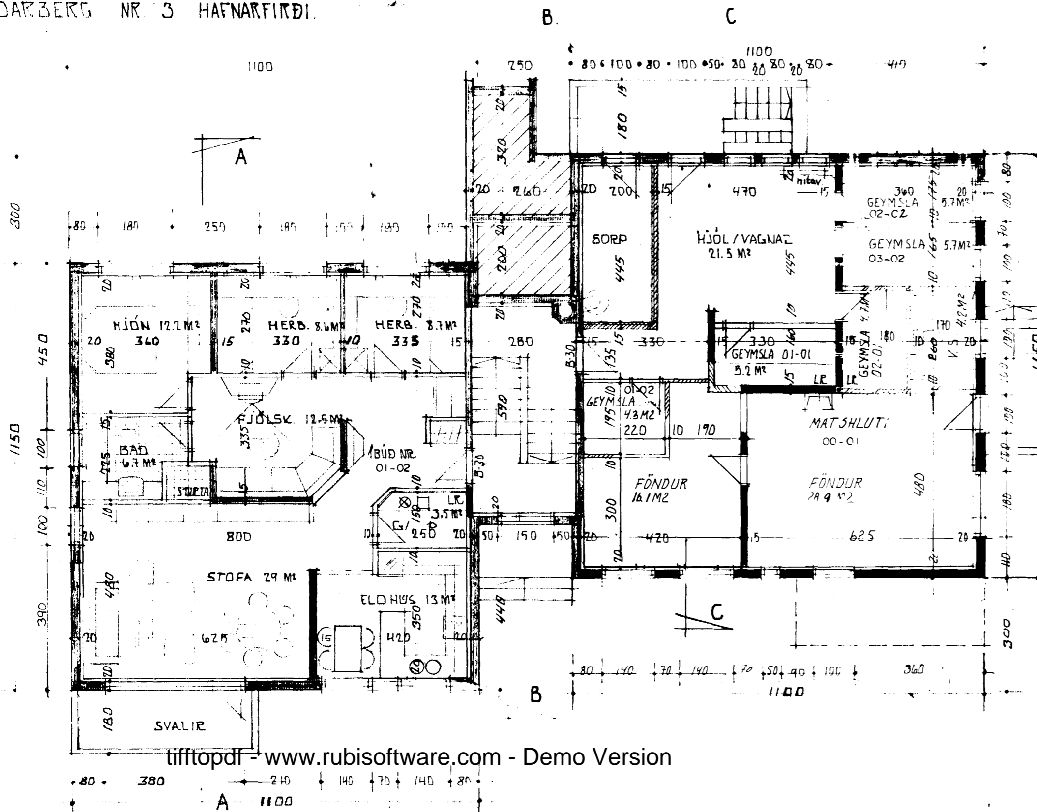
GRUNNMYND I. HÆÐ OG KJALLARI M. 1:100
