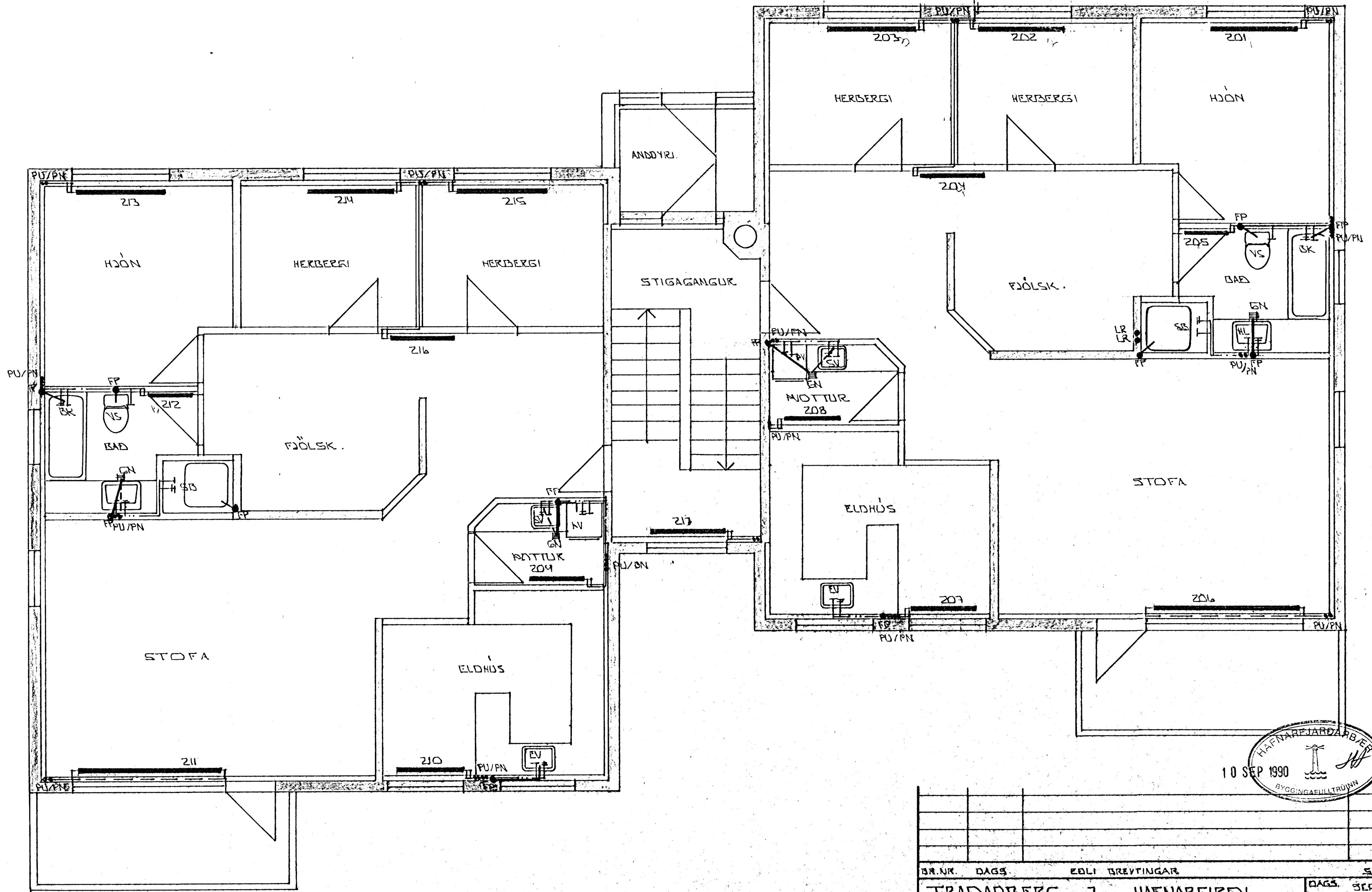
GRUNNMÝND 2. HÆÐ 1:20
