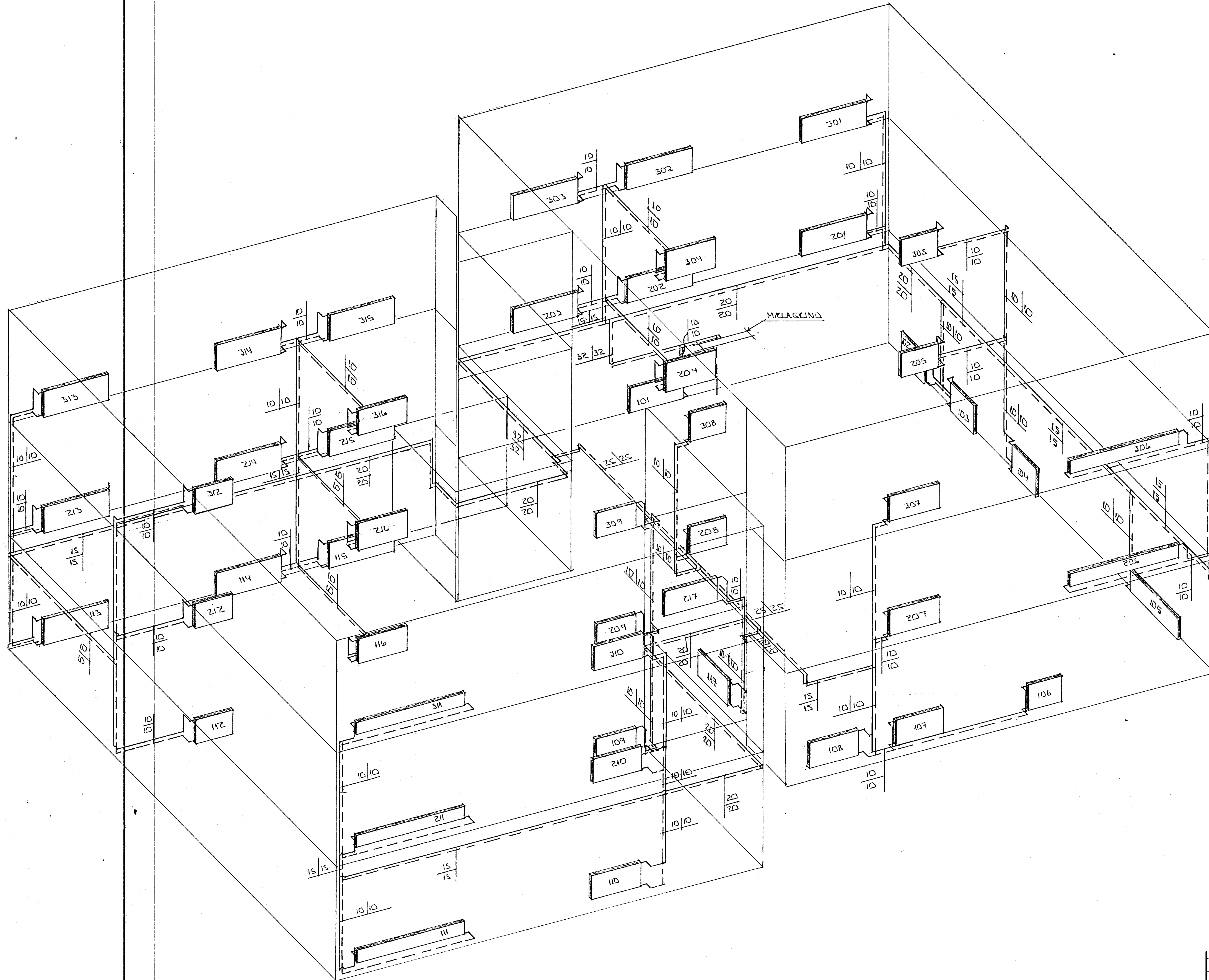
RÚMMYND HITLAGNA 1:50
