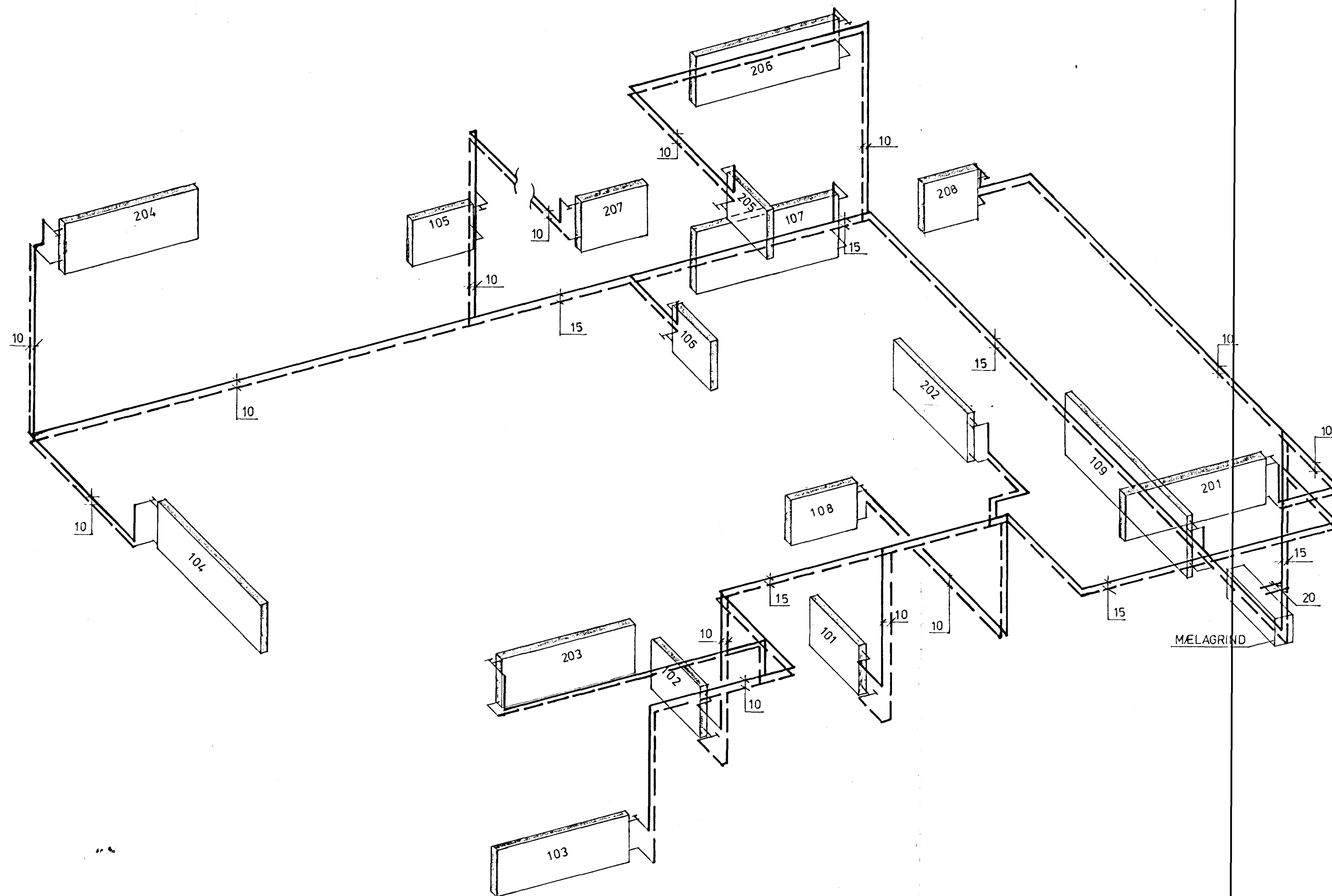
RÚMMYND ~ 1:50
