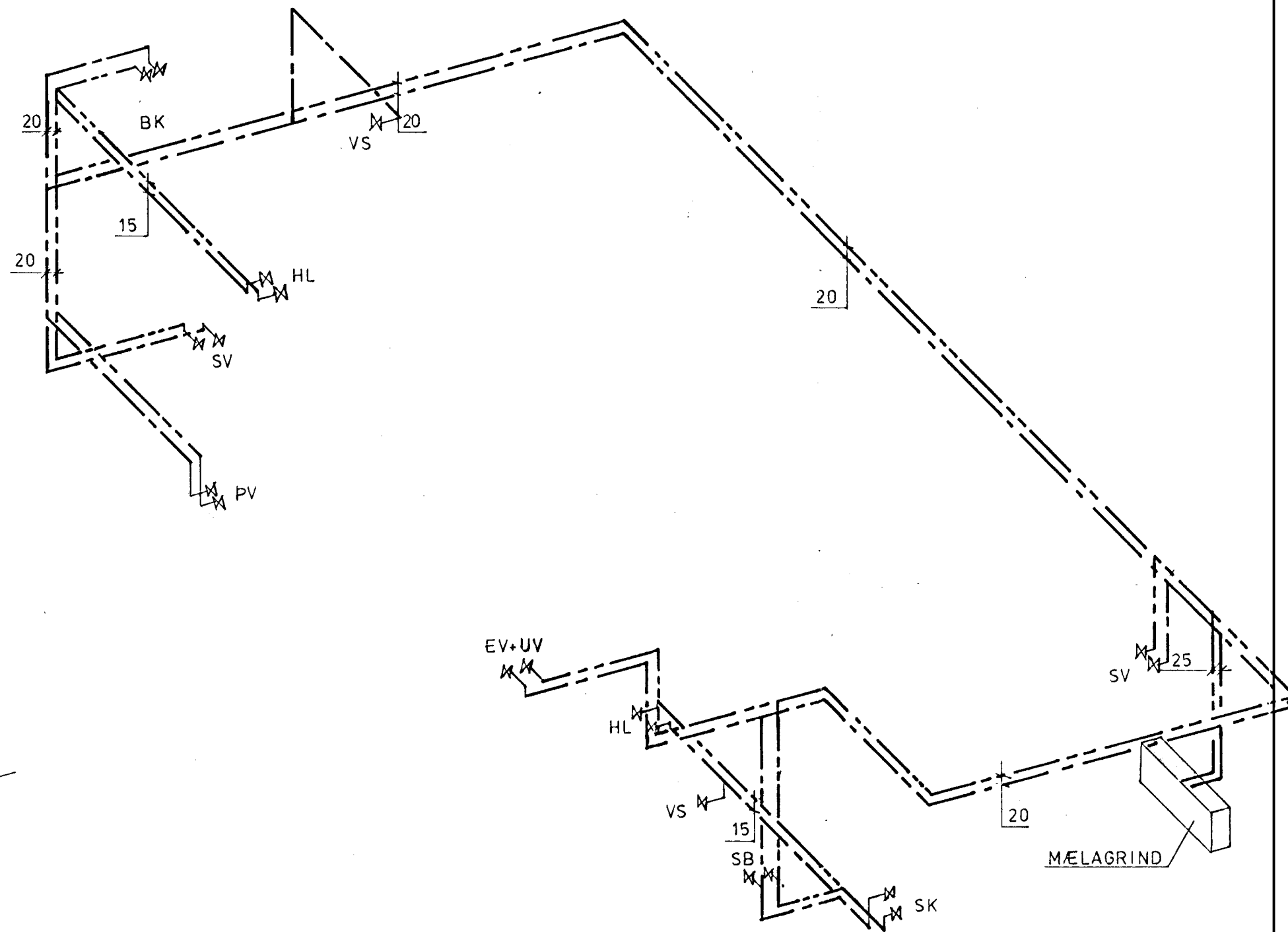
RÚMMYND VATNSLAGNA ~ 1 : 50
