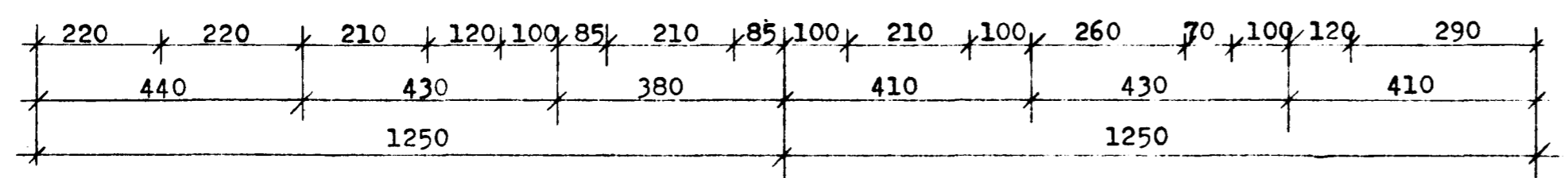
GRUNNMYND 2. HÆÐAR
