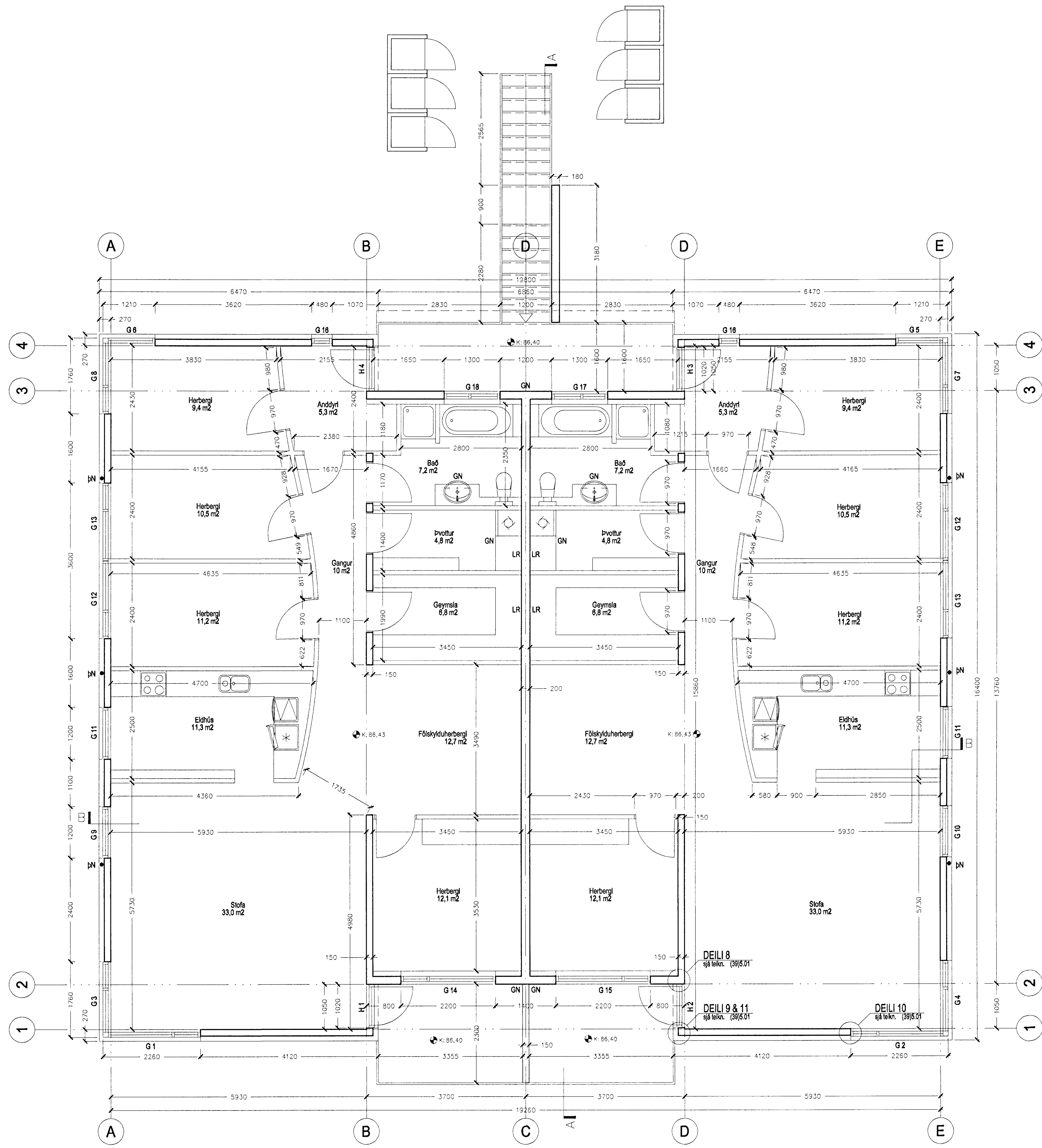
GRUNNMYND 2. HÆÐAR mkv. 1:50
