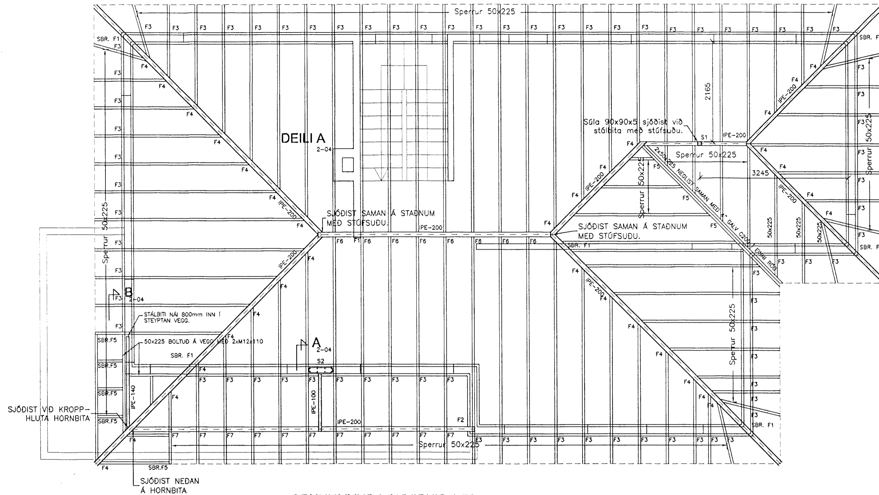
GRUNNMYND ÞAKVIRKIS 1:50
