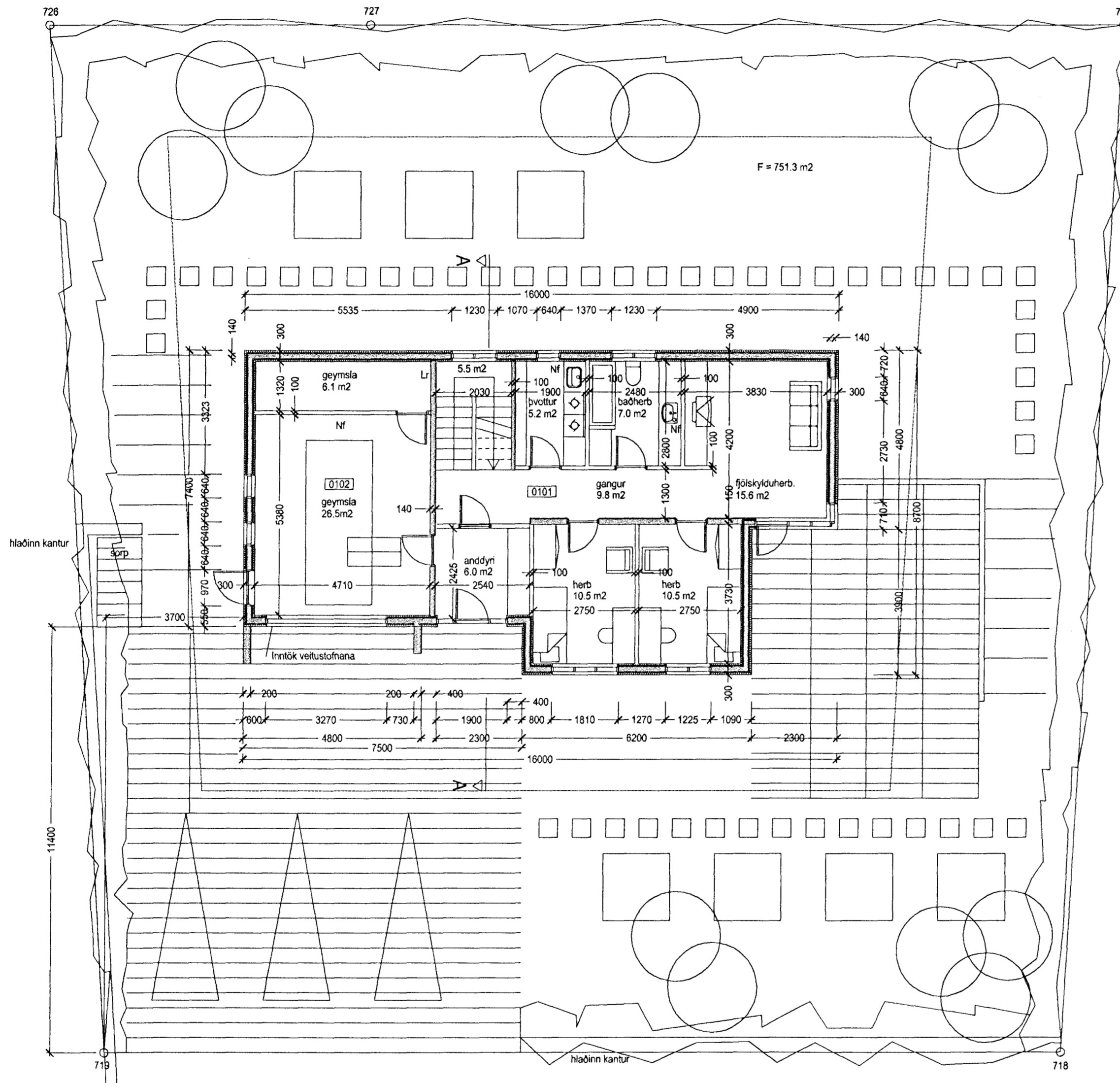
GRUNNMYND NEDRI HÆÐ 1 : 100
