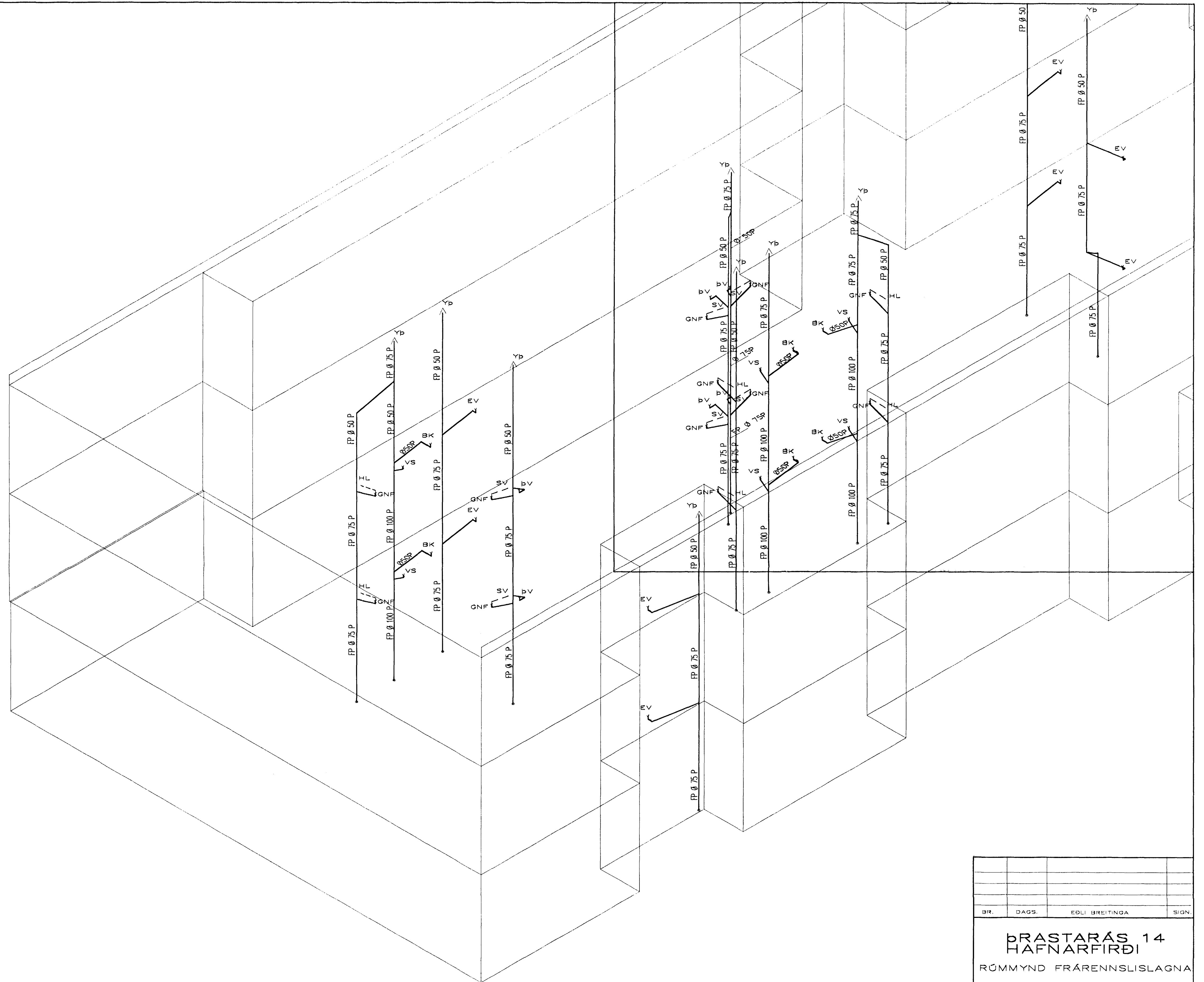
RÚMMYND FRÆRENNSLISLAGNA 1:50
