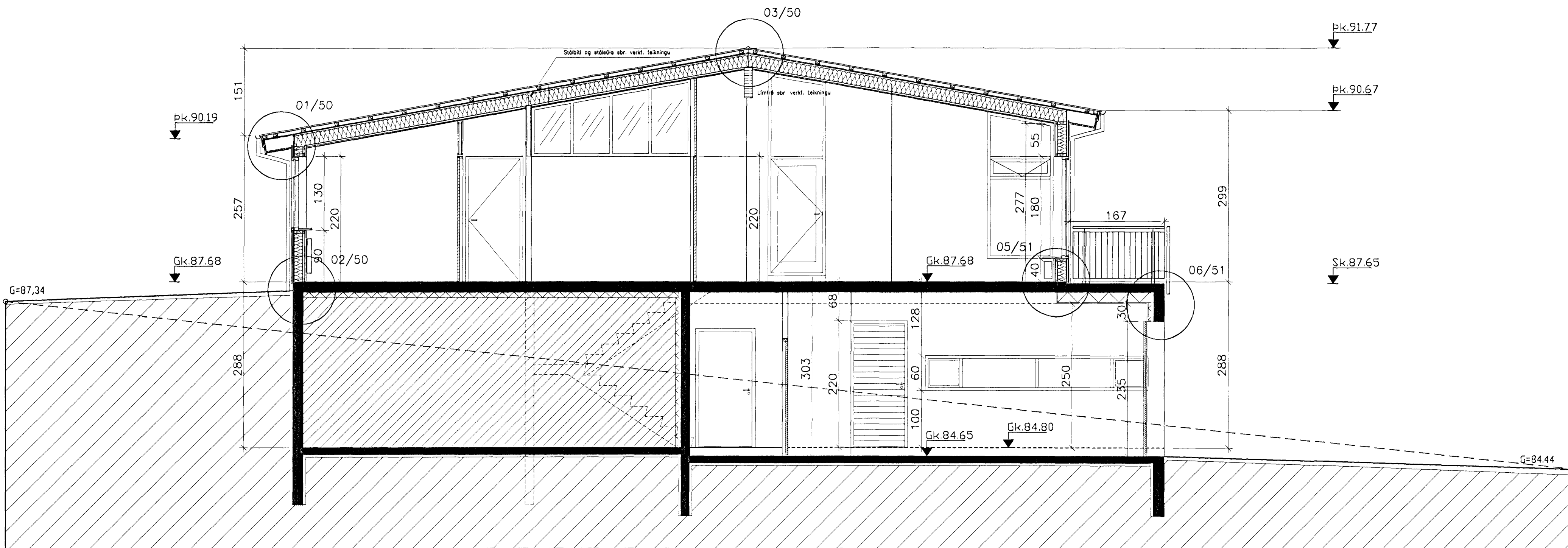
SNEIÐING A-A
