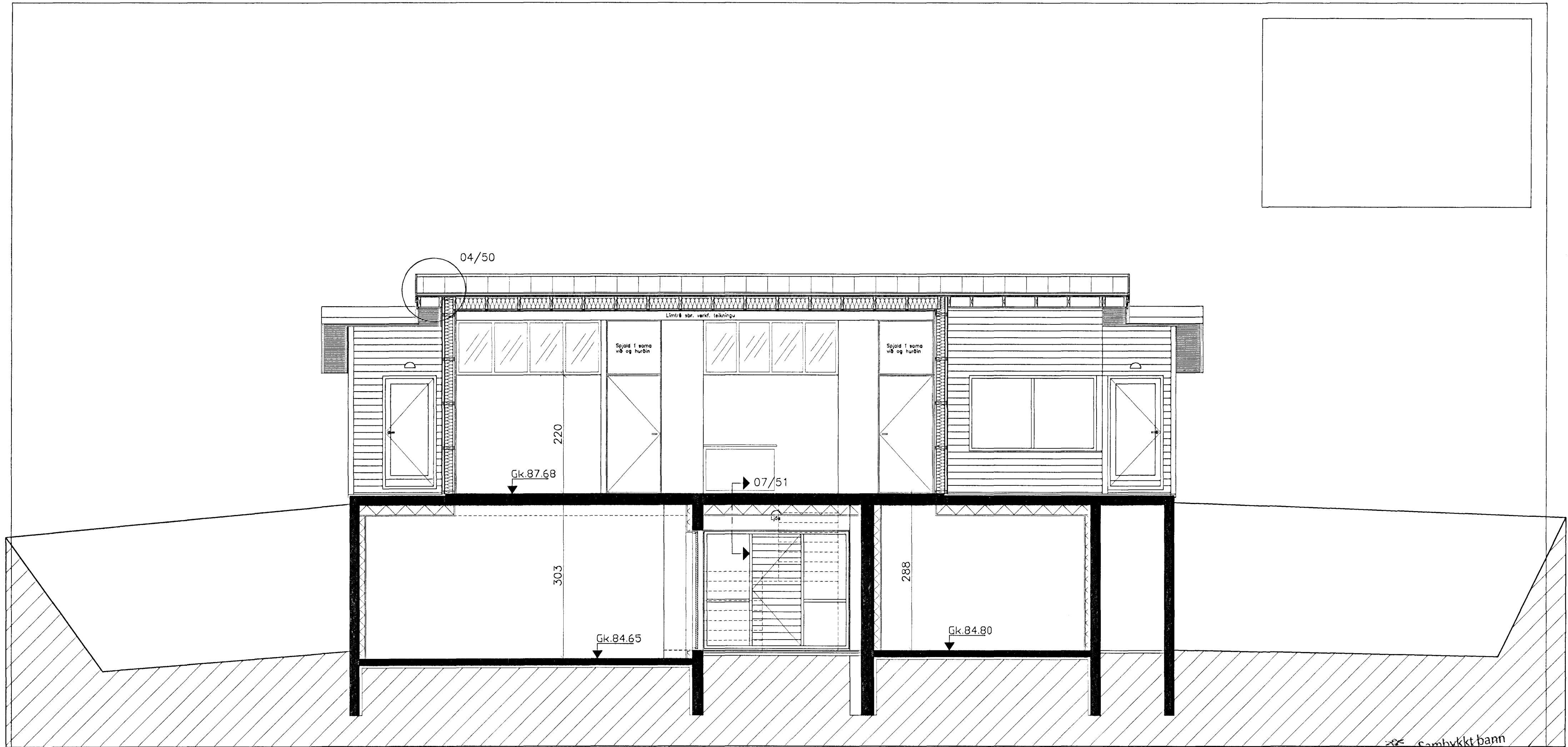
SNEIÐING B-B
