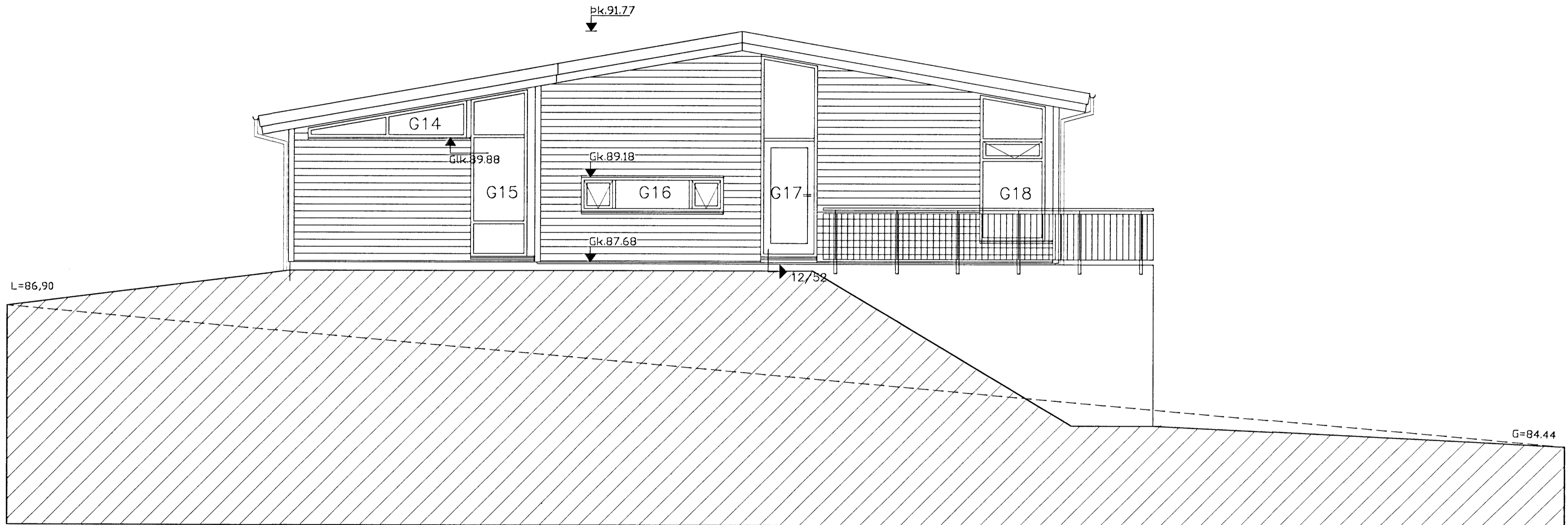
ÚTLIT N-V
