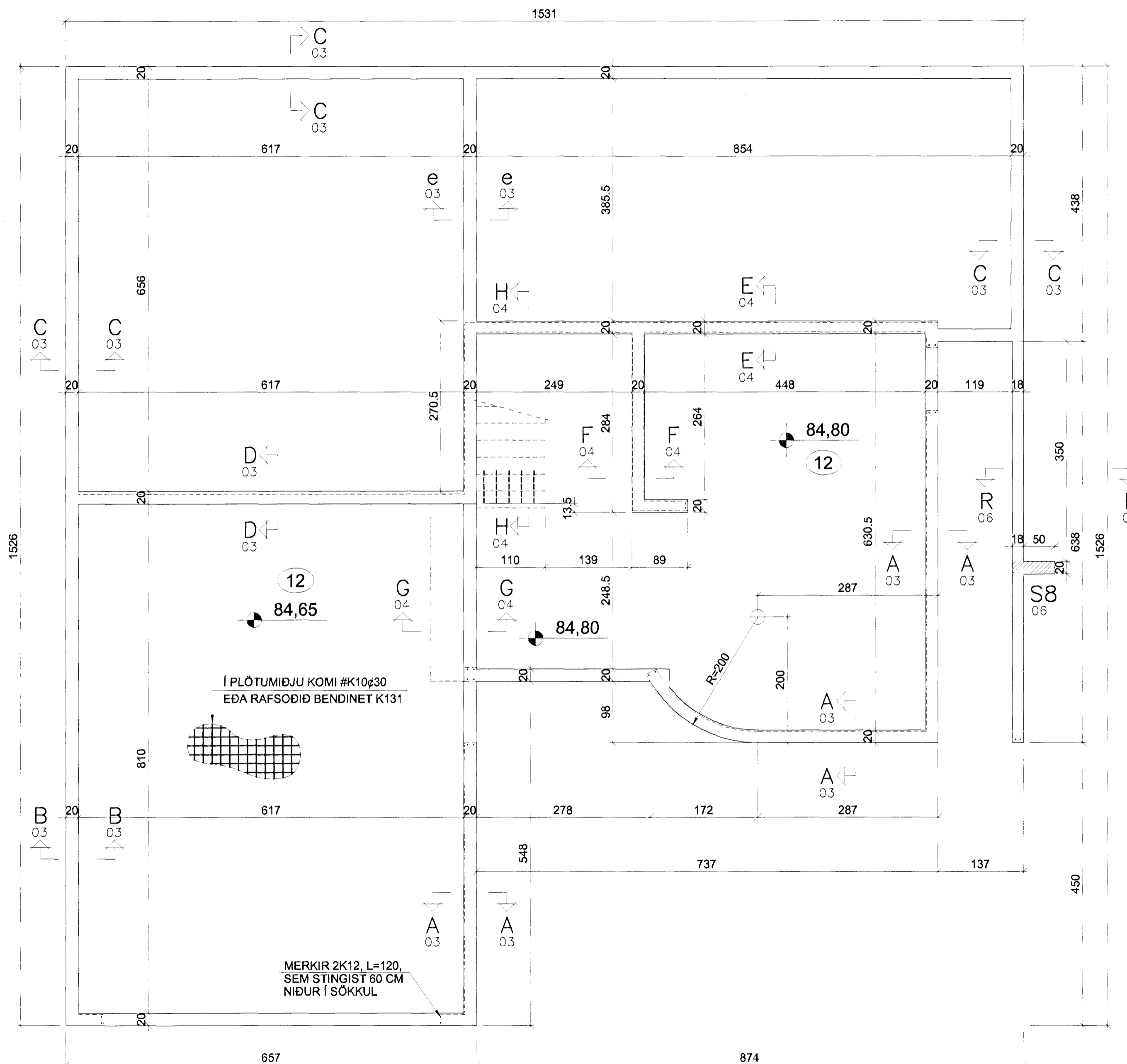
GRUNNMYND 1:50
