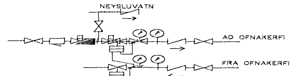
MÆLAGRIND HITAVEITU
