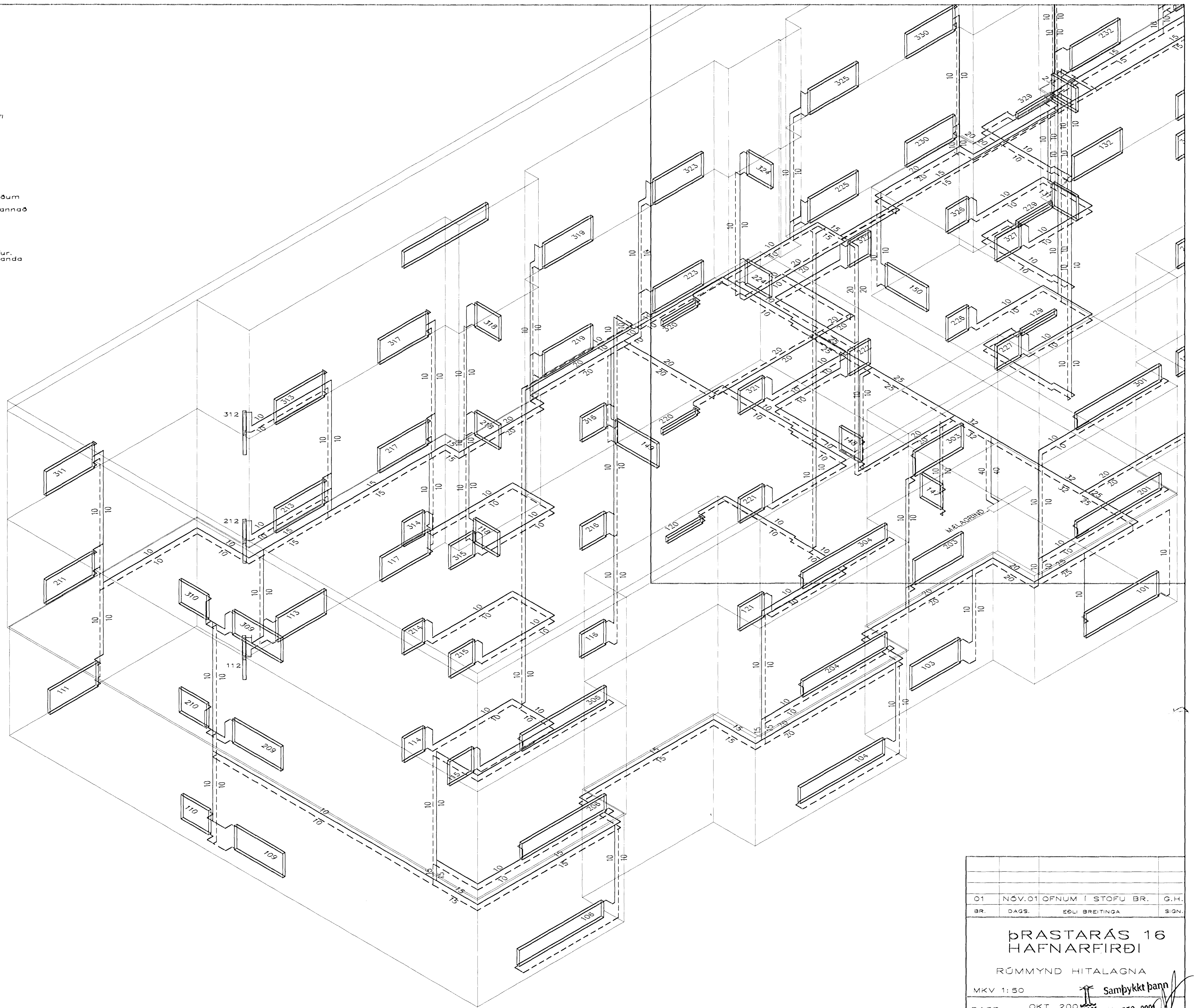
RÜMMYND HITALAGNA 1:50
