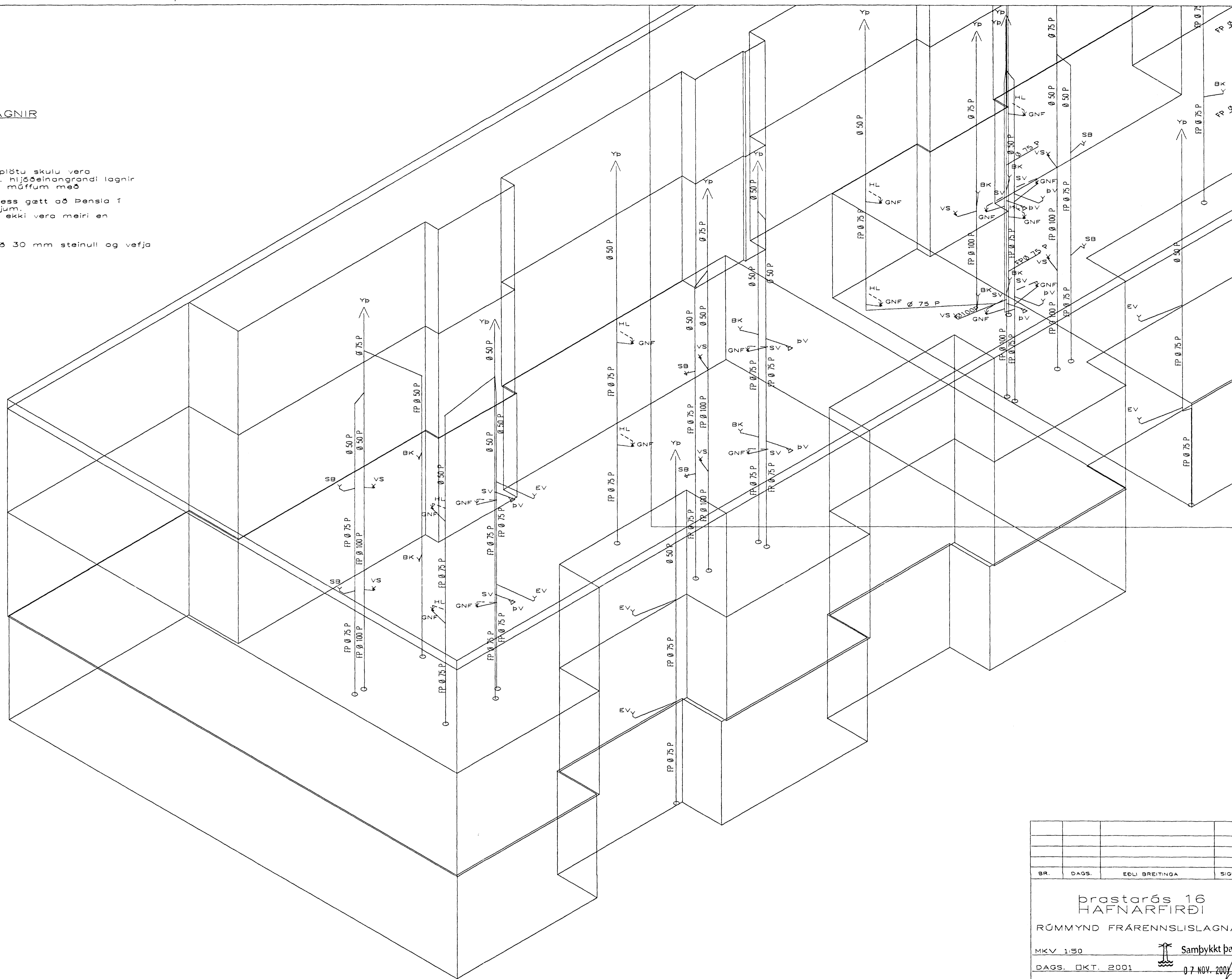
RÚMMYND FRÁRENNSLISLAGNA 1:50
