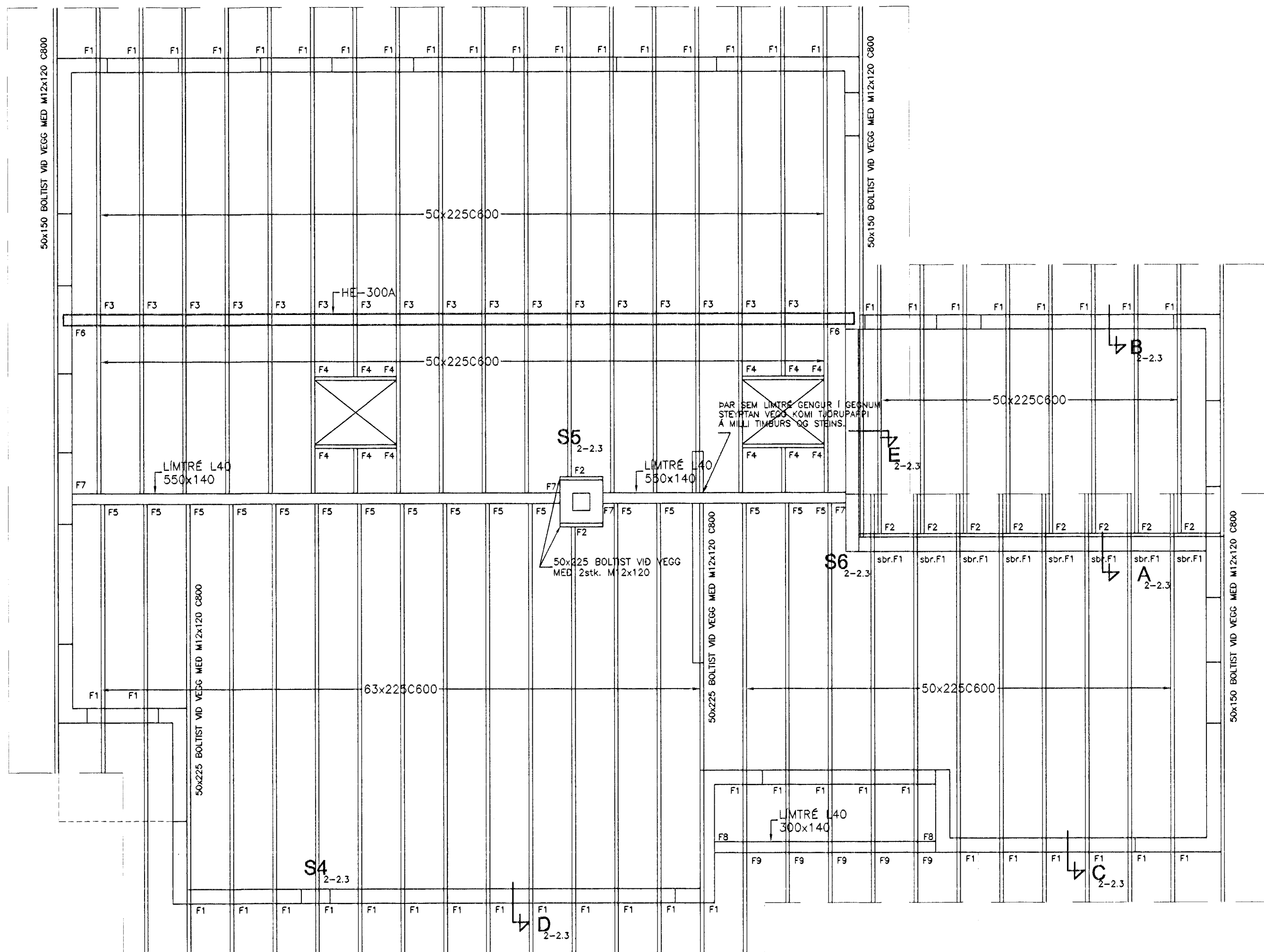
GRUNNMYND ÞAKS 1:50 FESTINGAR ERU SÝNDAR Á BLADI 2-2.2
