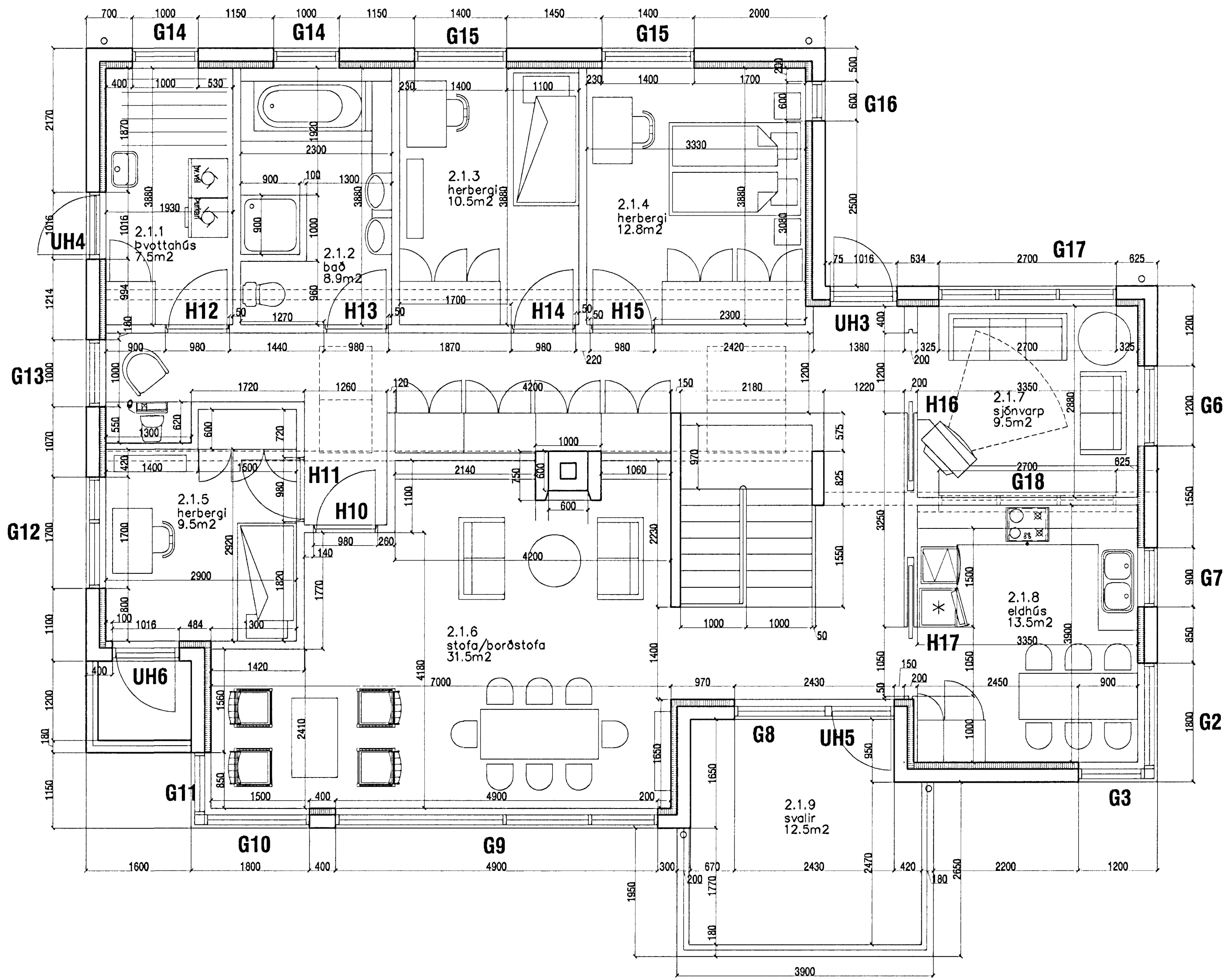
GRUNNMYND 2. HÆÐAR mkv. 1:50
