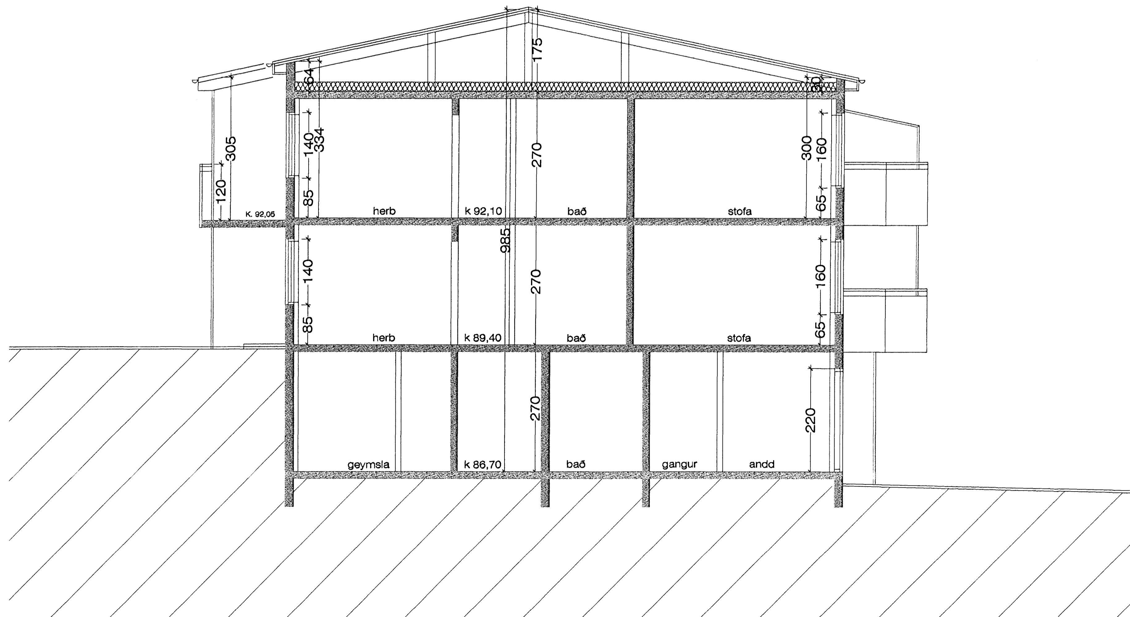
SNEIÐING B - B M 1 : 50
