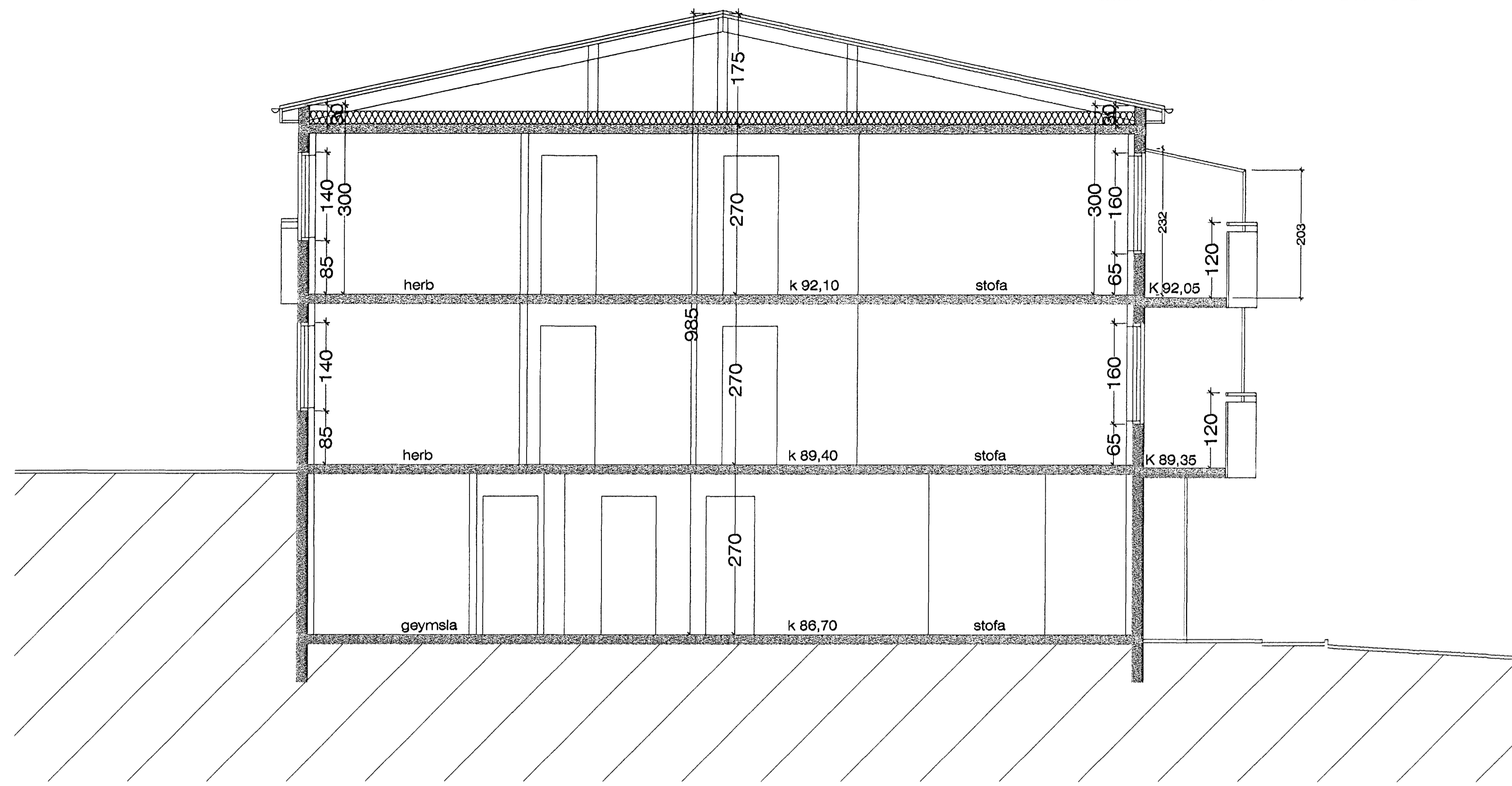
SNEIÐING A - A M 1 : 50
