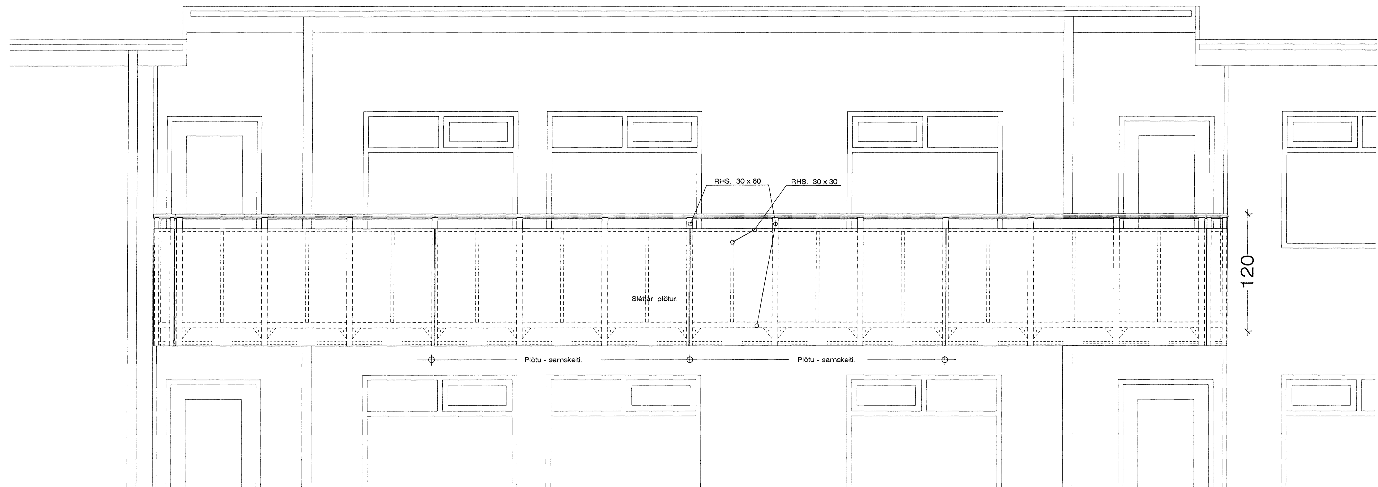
Séð framaná gangsvalahandrið. 1:20
