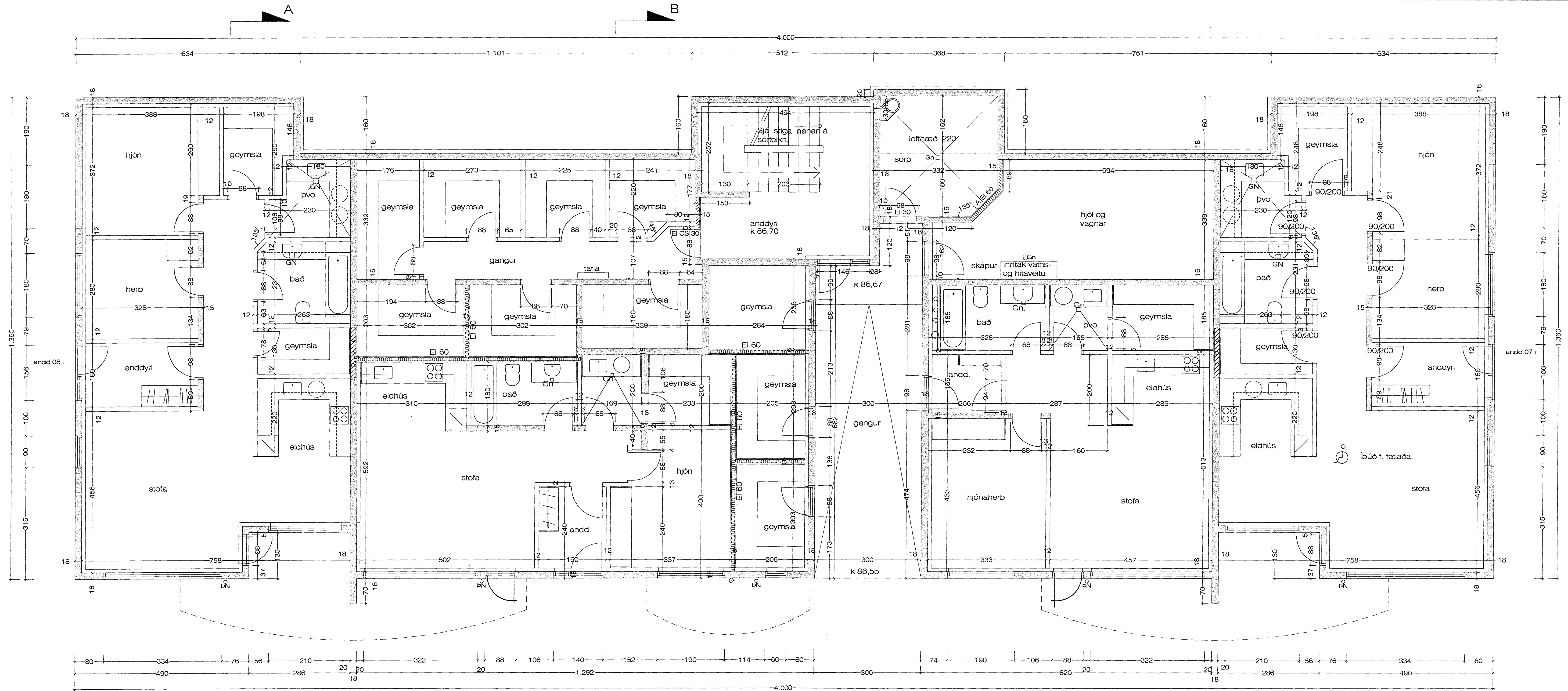
GRUNNMYND 1. HÆÐ M 1 : 50
