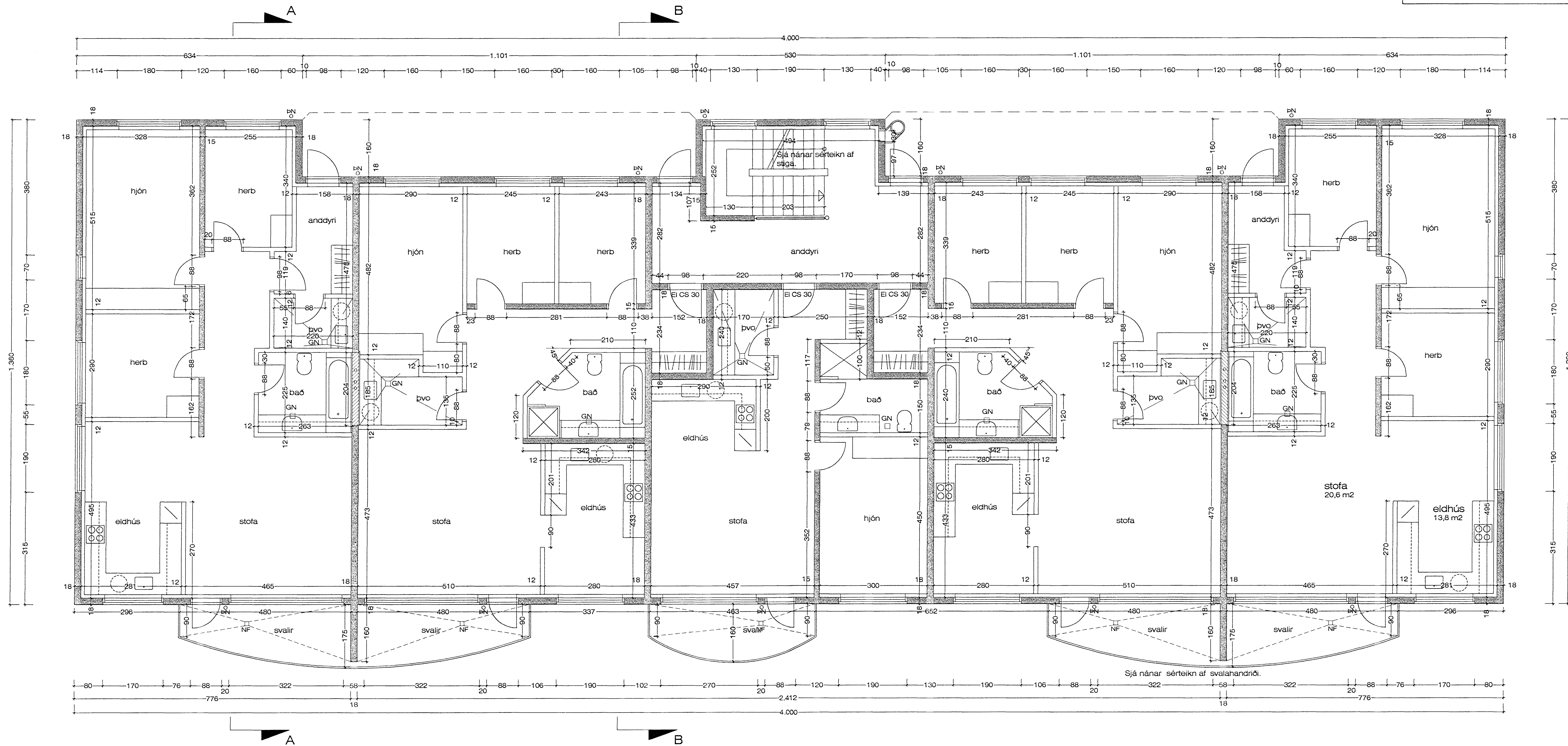
GRUNNMYND 2. HÆÐ M 1 : 50
