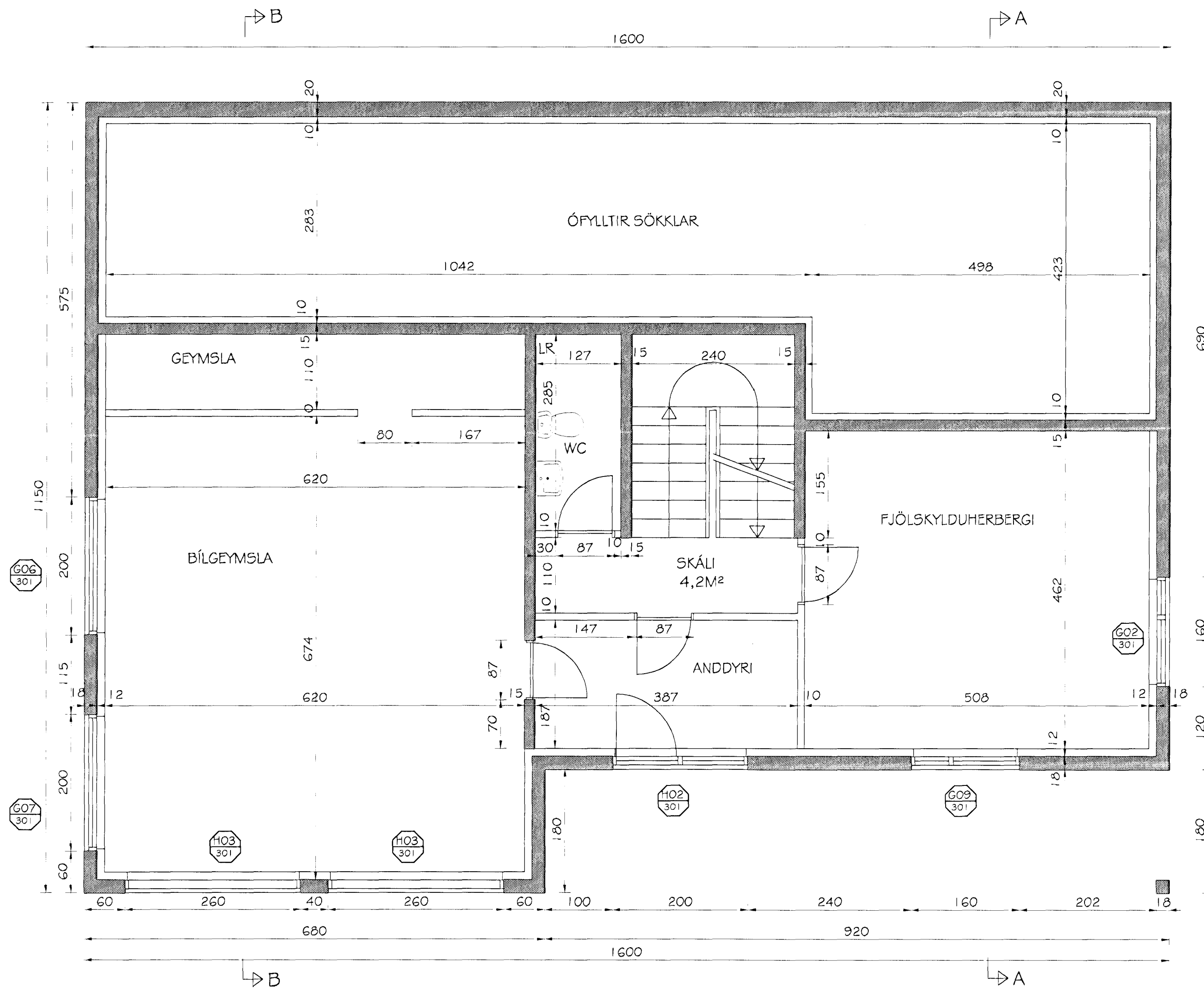
GRUNNMYND NEDRI HÆÐAR MKV. 1:50
