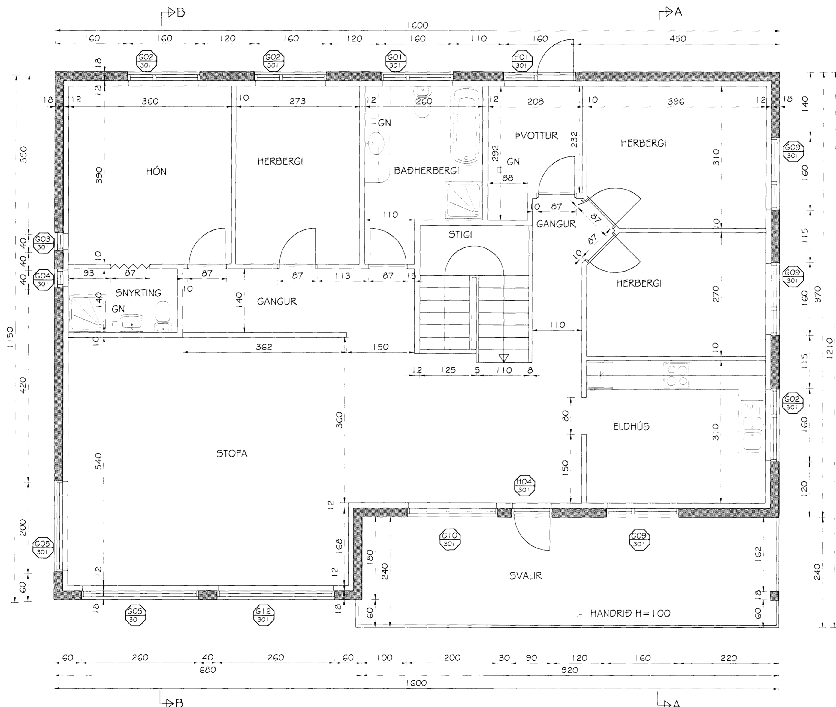
GRUNNMYND EFRI HÆÐAR MKV. 1:50
