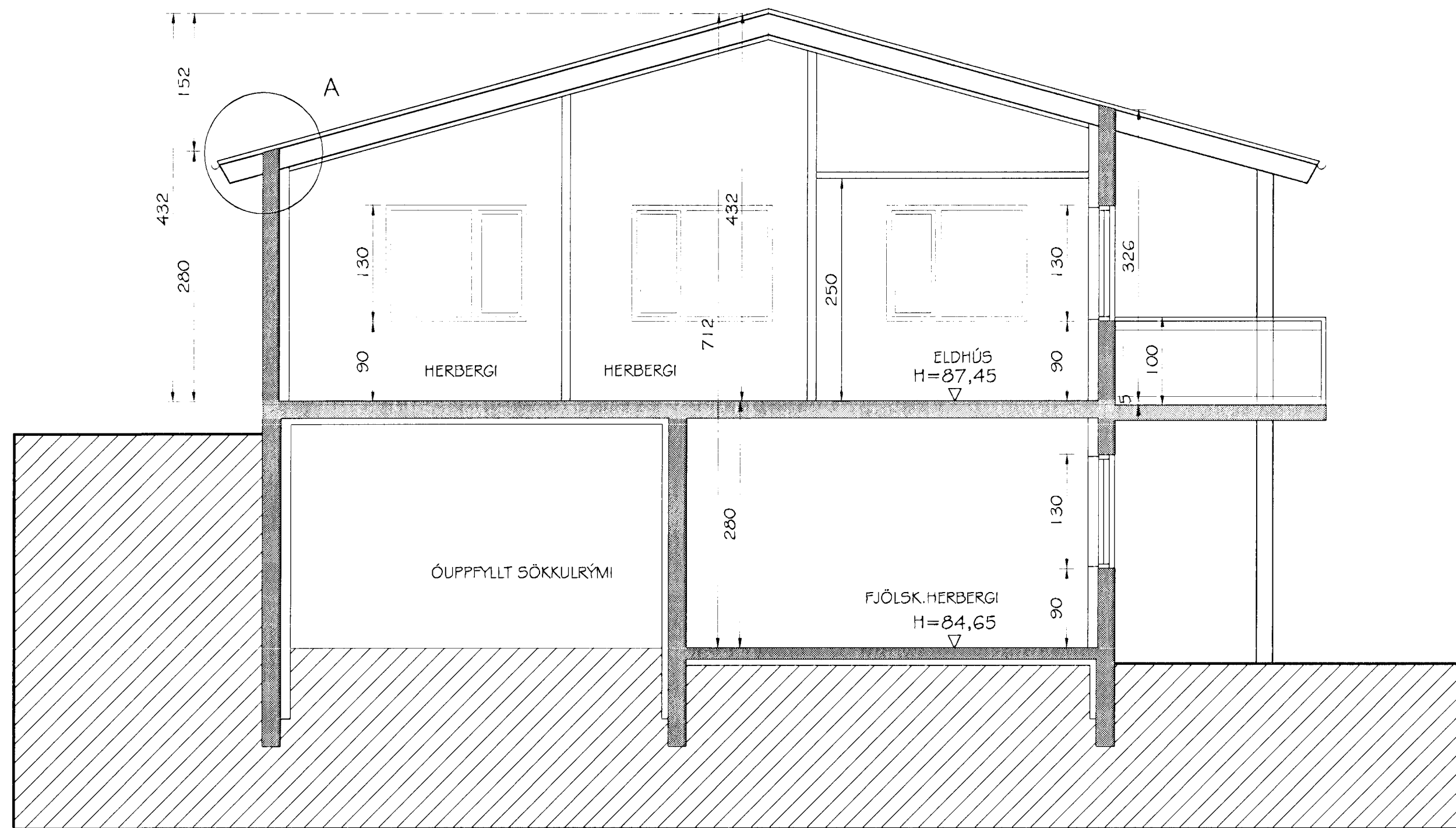
SNID A-A MKV. 1:50
