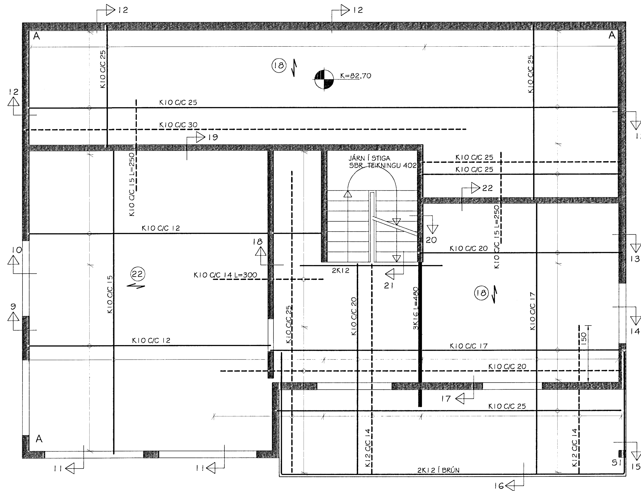
JÁRN Í PLÖTU YFIR NEDRI HÆÐ - GRUNNMYND MKV. 1:50
