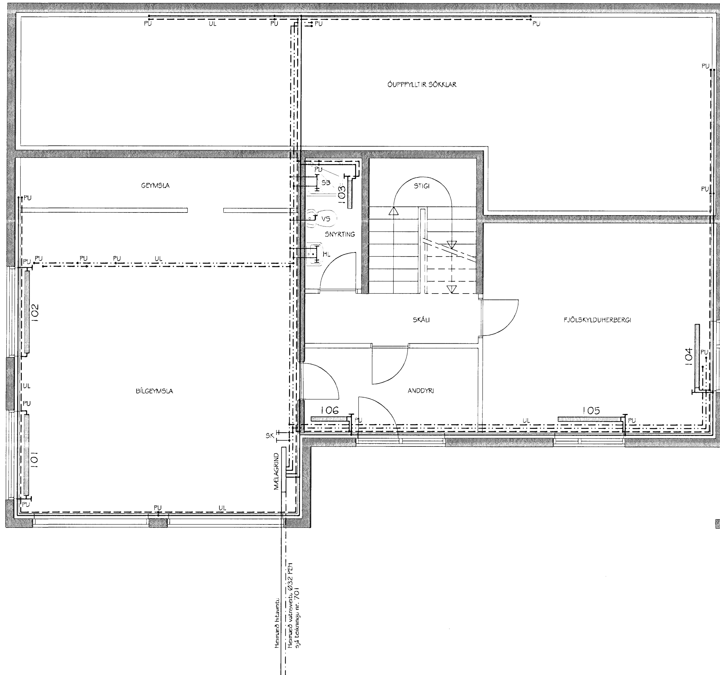
HITA- OG NEYSLUVATNSLAGNIR GRUNNMYND NEDRI HÆÐAR MKV. 1:50
