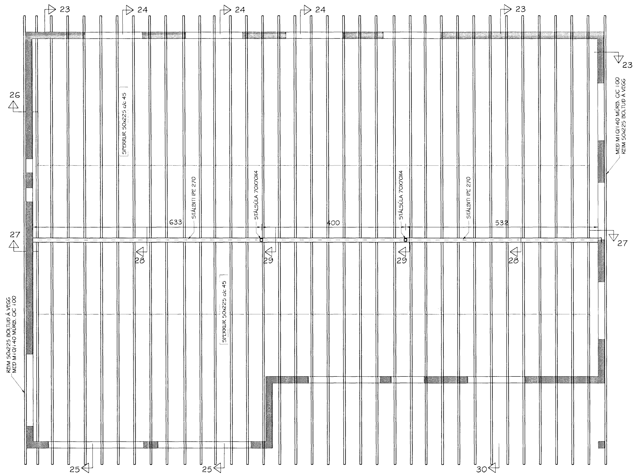
GRUNNMYND ÞAKVIÐA MKV. 1:50
