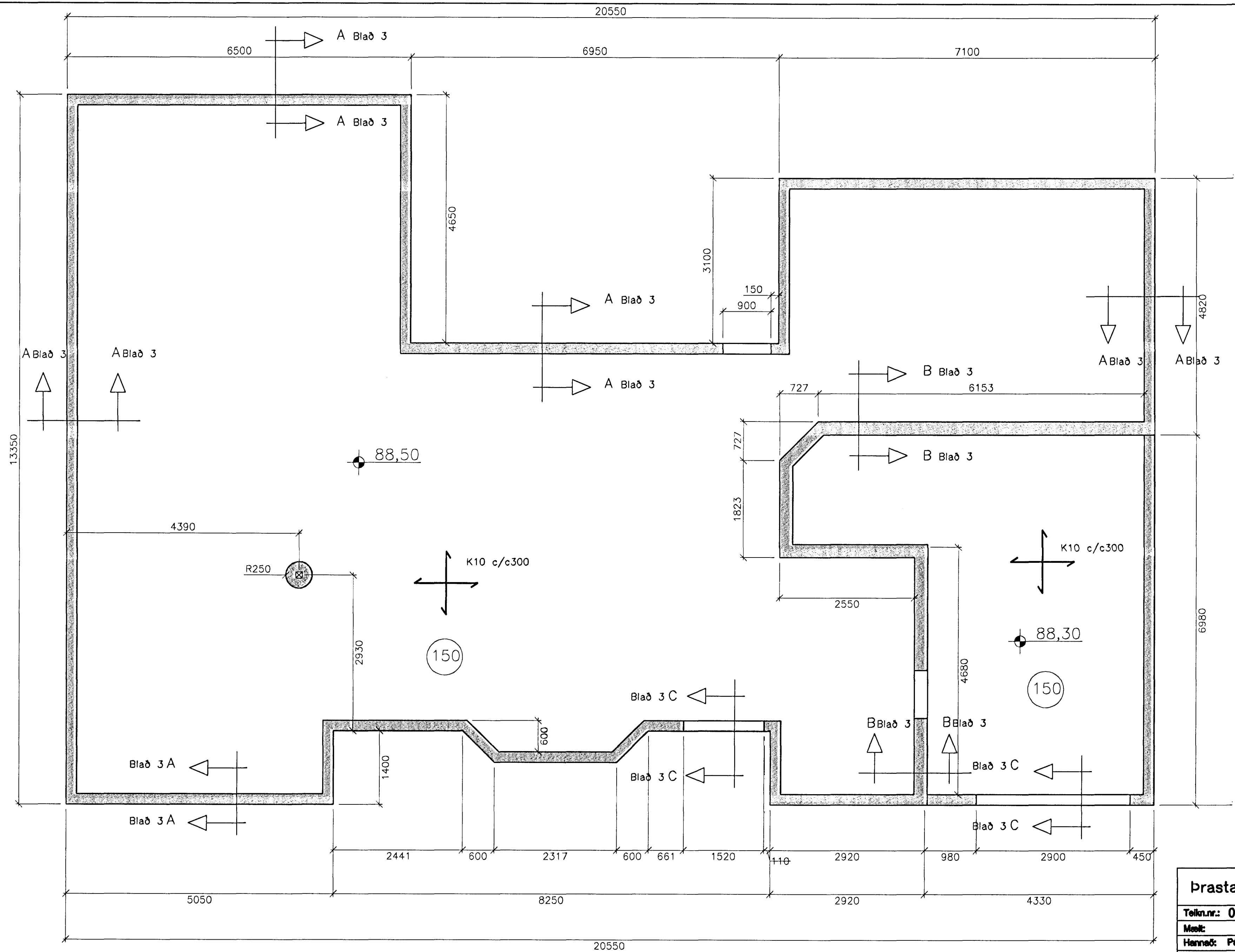
Grunnmynd sökkla 1:50
