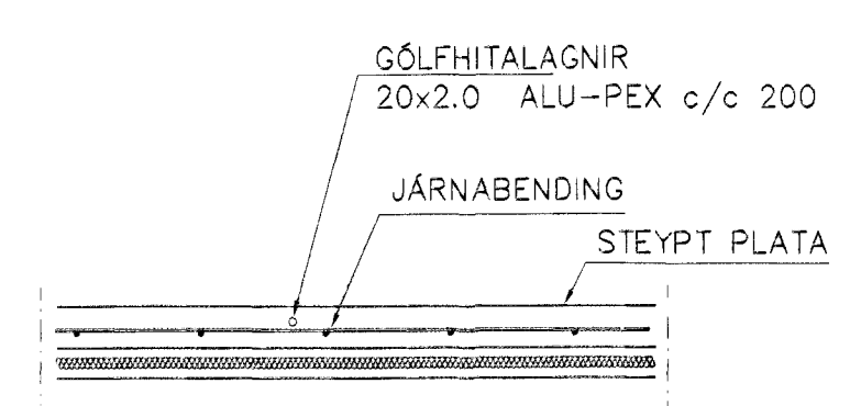
LAGNIR, SNÍÐ, 1:20
