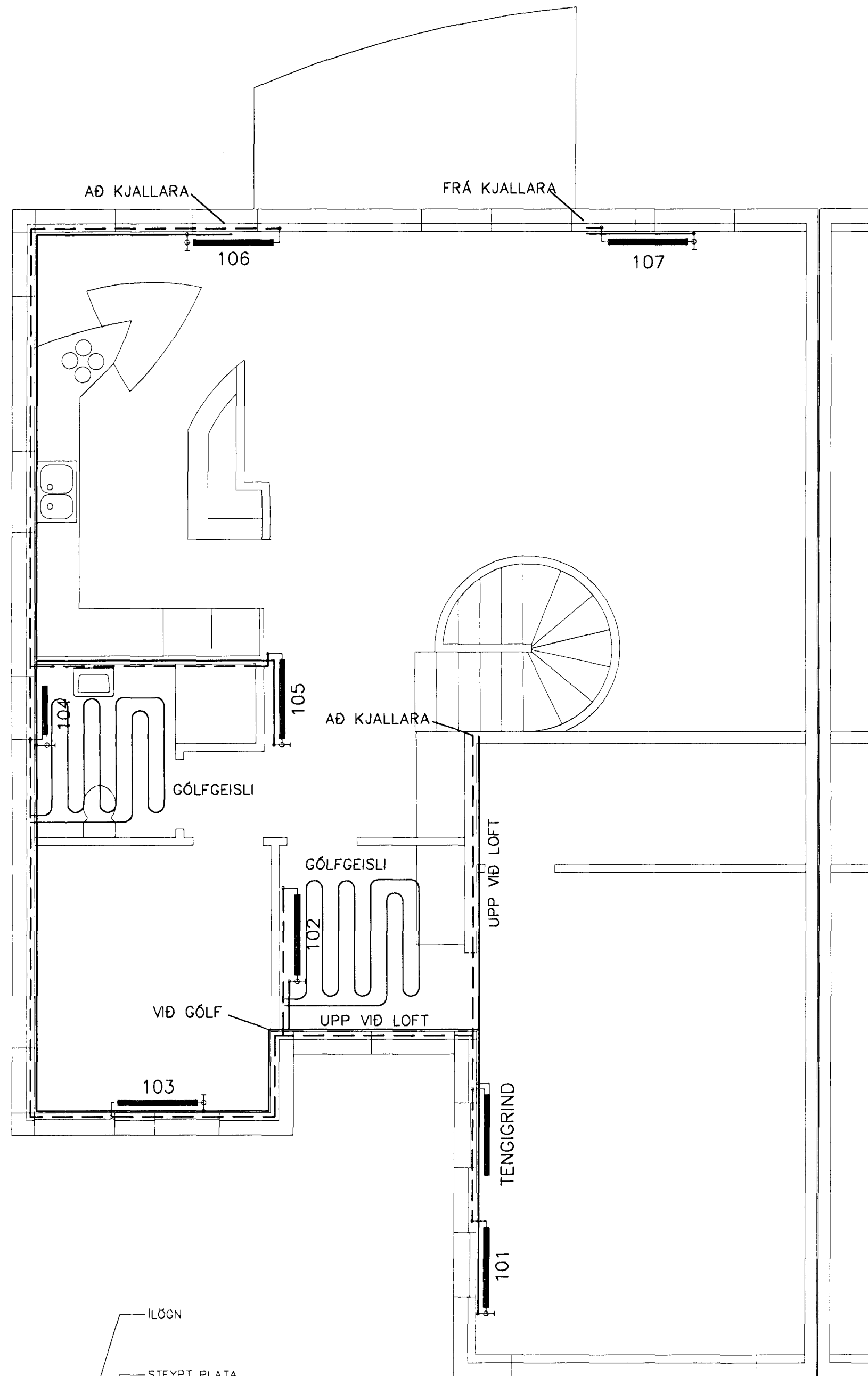
GRUNNMYND 1:50
