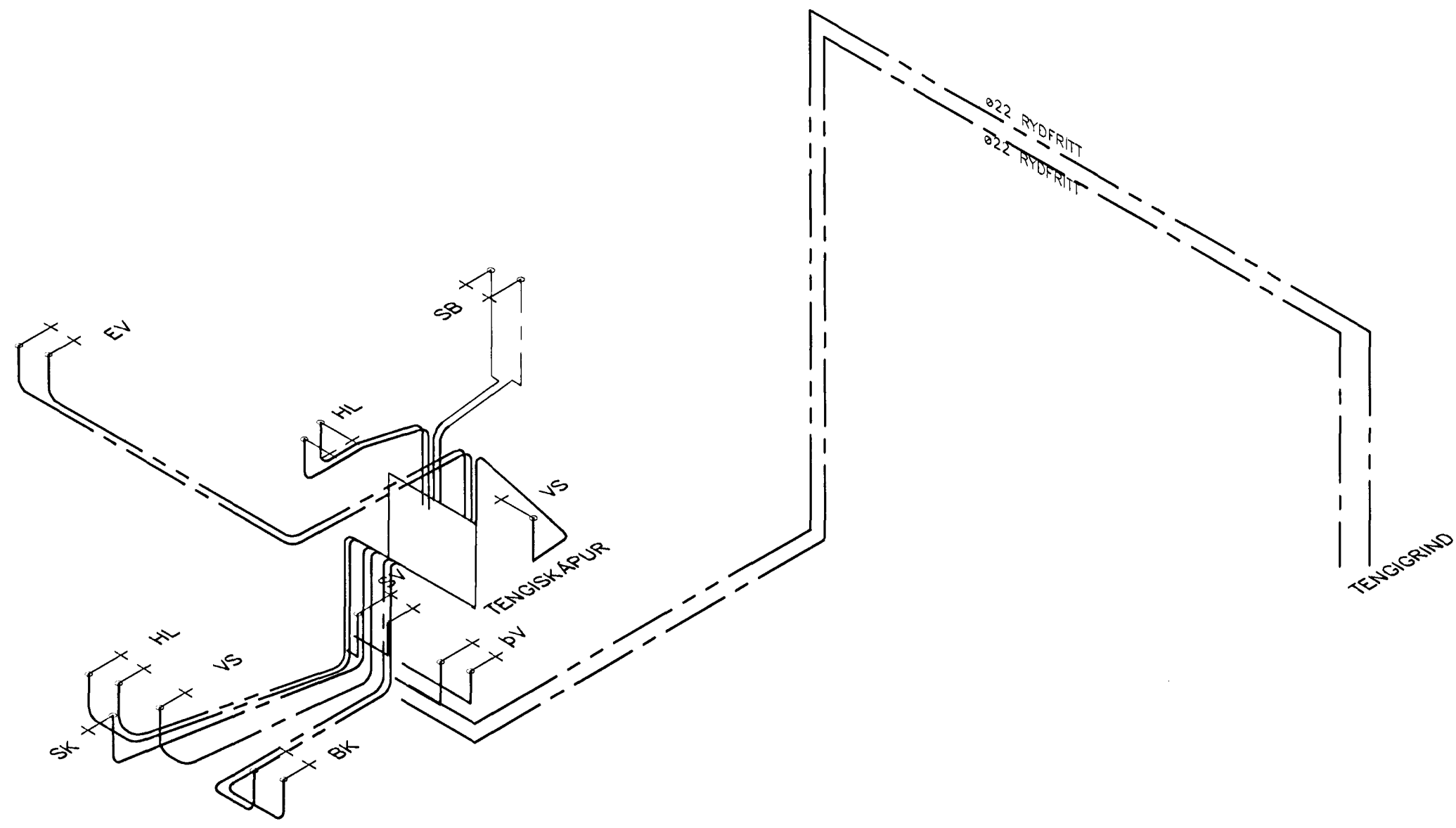
GRUNNMYND 1:50
