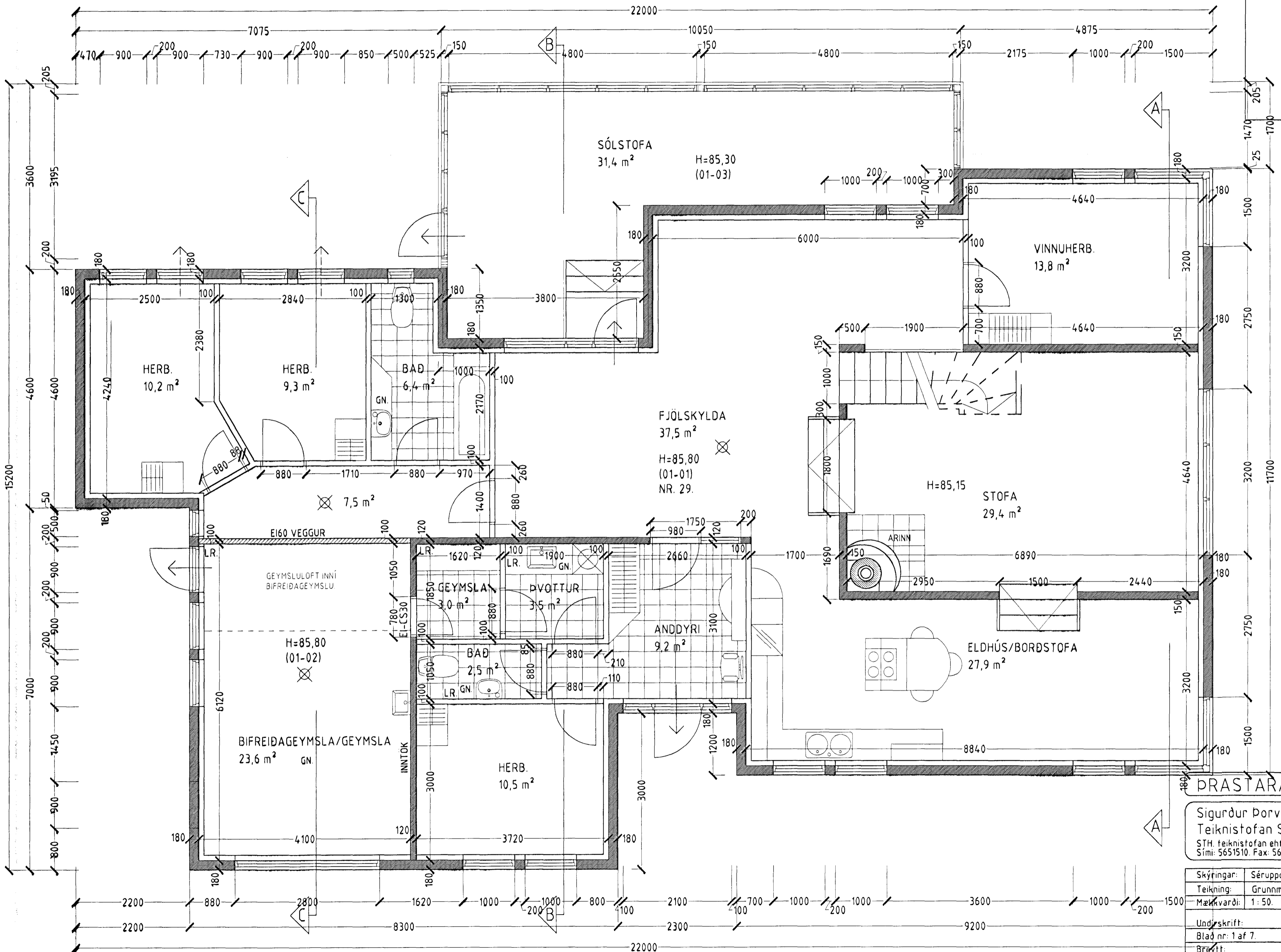
GRUNNMYND 1 HÆÐ MKV. 1:50.
